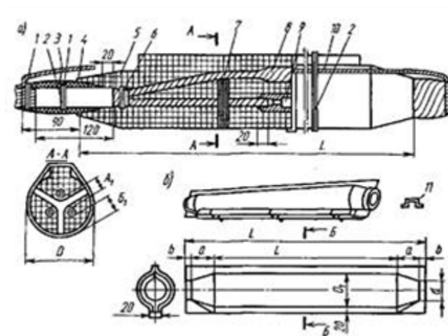
Рисунок 4.6 - Эпоксидная соединительная муфта на напряжение 6 и 10 кВ:
