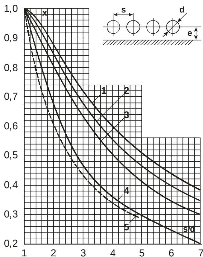
Рис. 3.2. Угловые коэффициенты однорядного гладкотрубного экрана 1 – с учетом излучения обмуровки при e \geq 1,4d ; 2 – то же при e=0,8d ; 3 – то же при e=0,5d ; 4 – то же при e=0 ; 5 – без учета излучения обмуровки при e \geq 0,5d .
