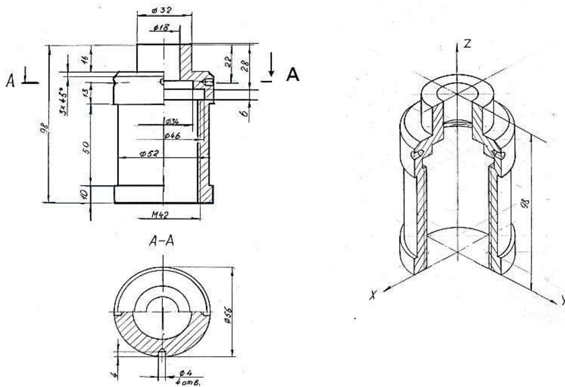
Рисунок 5 Вариант 5 (деталь Стакан)
