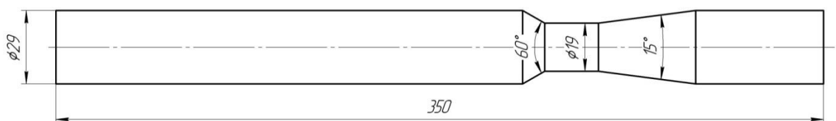
Рисунок 3 – Канал с конфузorno-диффузорной вставкой
