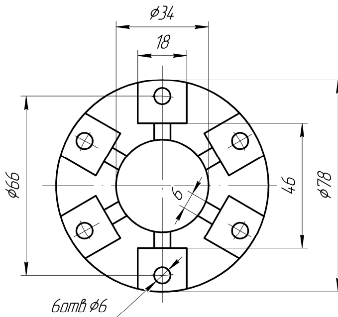
Диск
