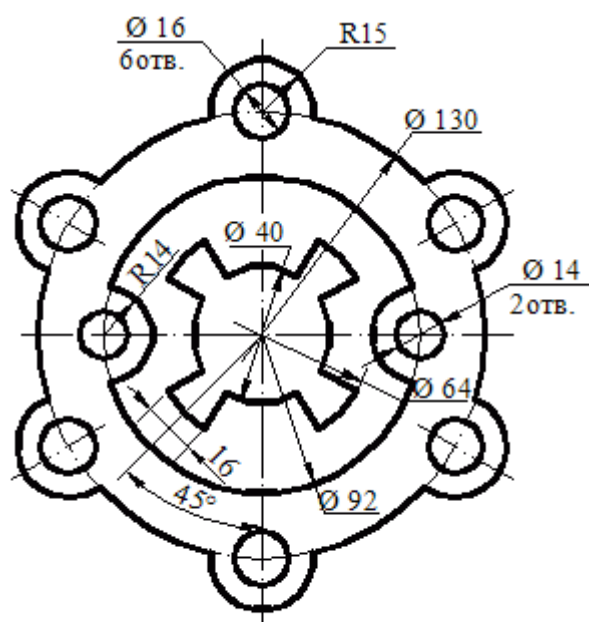
Крышка
