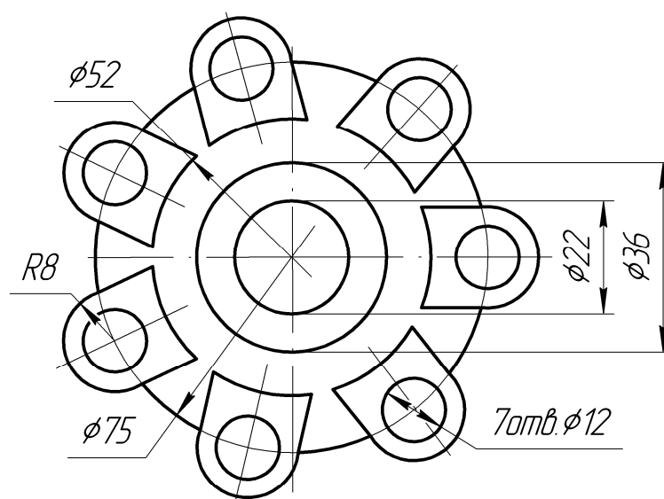
Крышка
