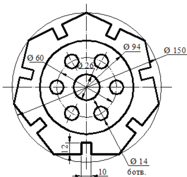
Пластина
