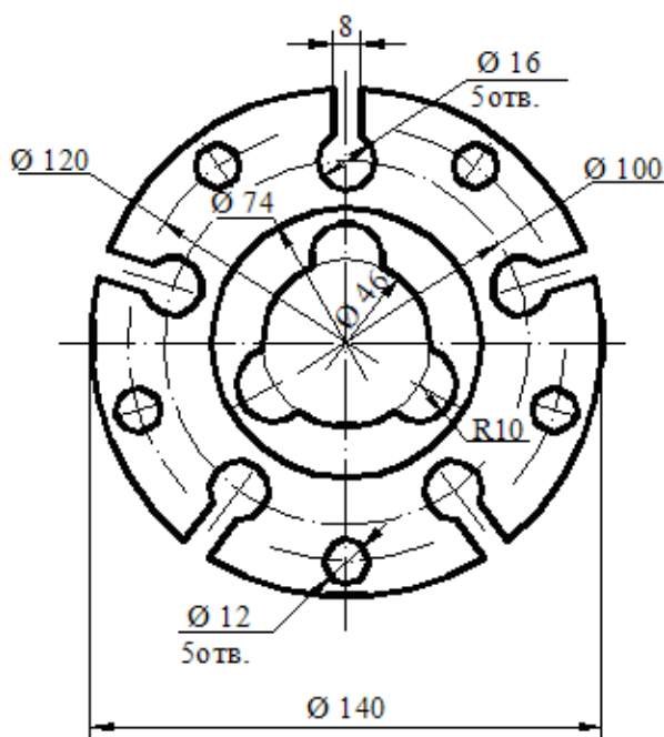
Прокладка
