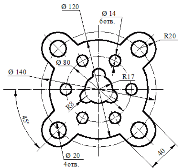
Фланец
