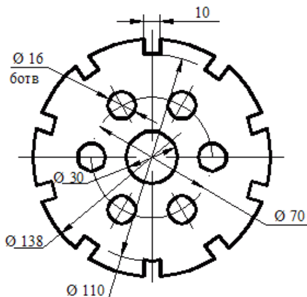
Прокладка
