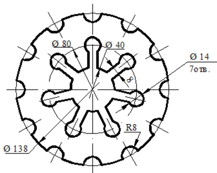
Прокладка
