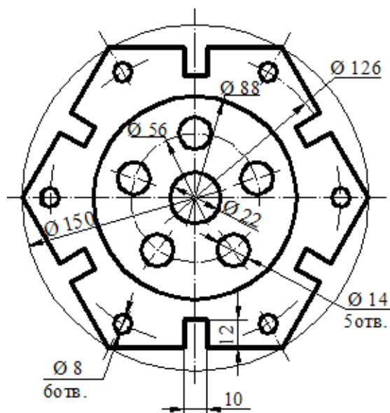
Пластина
