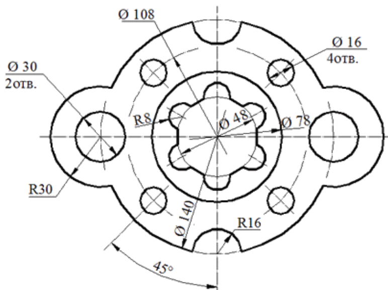
Крышка
