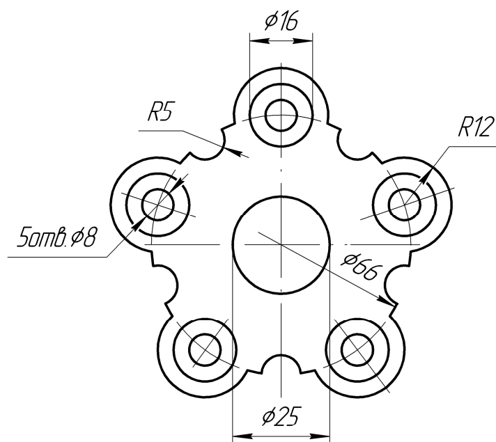
Прокладка
