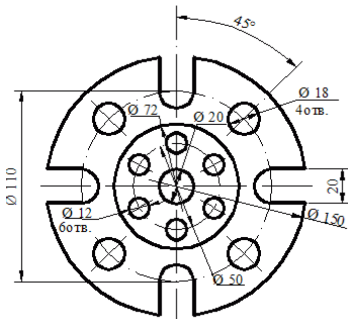
Фланец
