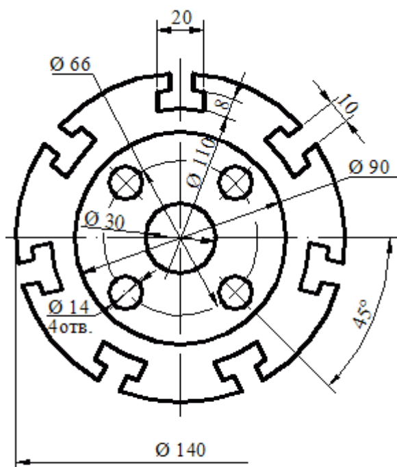
Пластина
