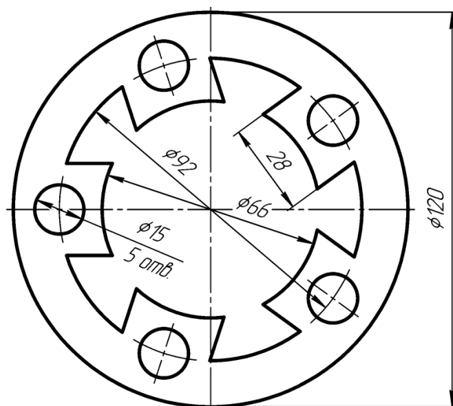
Прокладка
