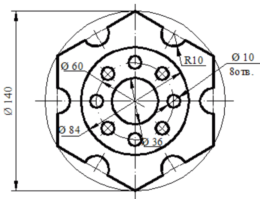
Пластина
