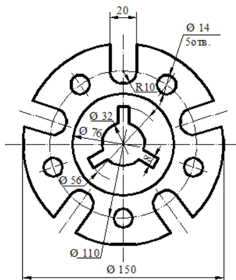
Фланец
