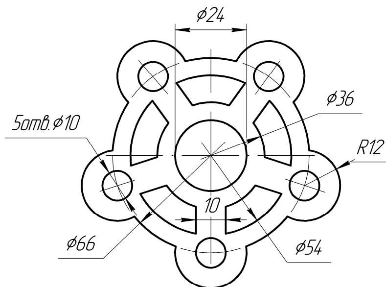
Прокладка
