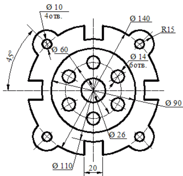
Крышка
