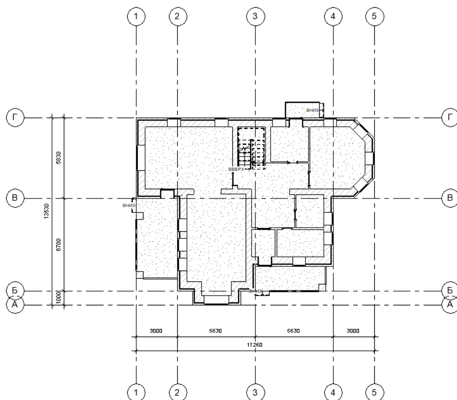
Рисунок 2 - План первого этажа
