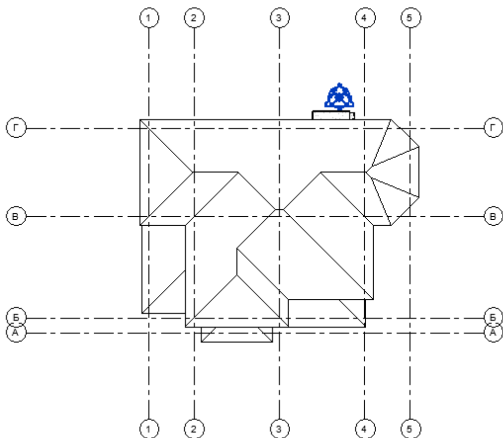
Рисунок 4 - План кровли
