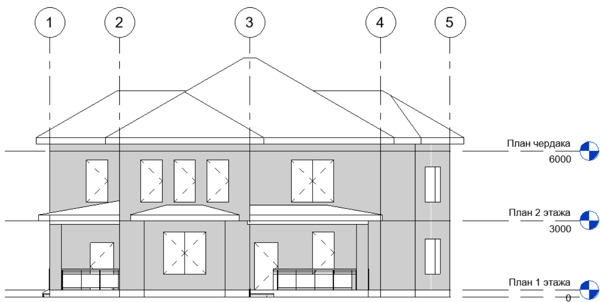
Рисунок 8 - Южный фасад
