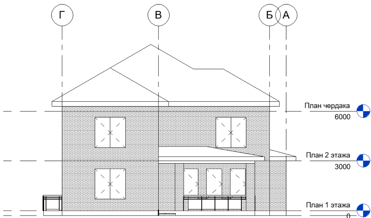
Рисунок 6 - Западный фасад
