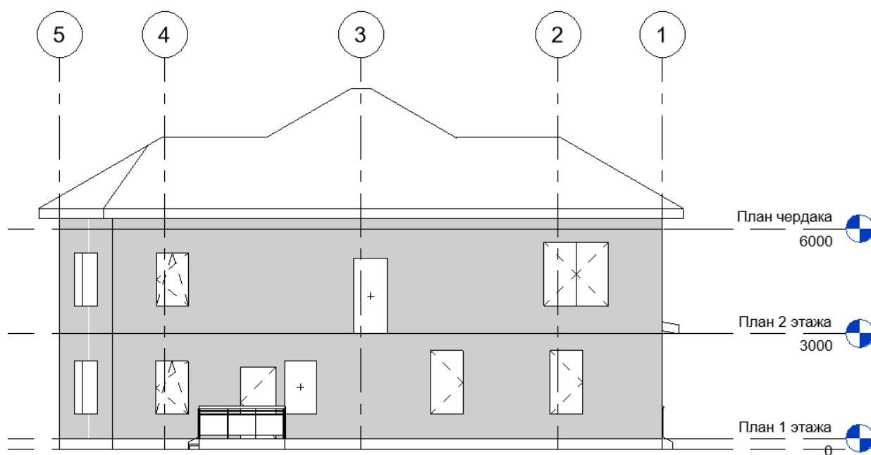
Рисунок 7 - Северный фасад
