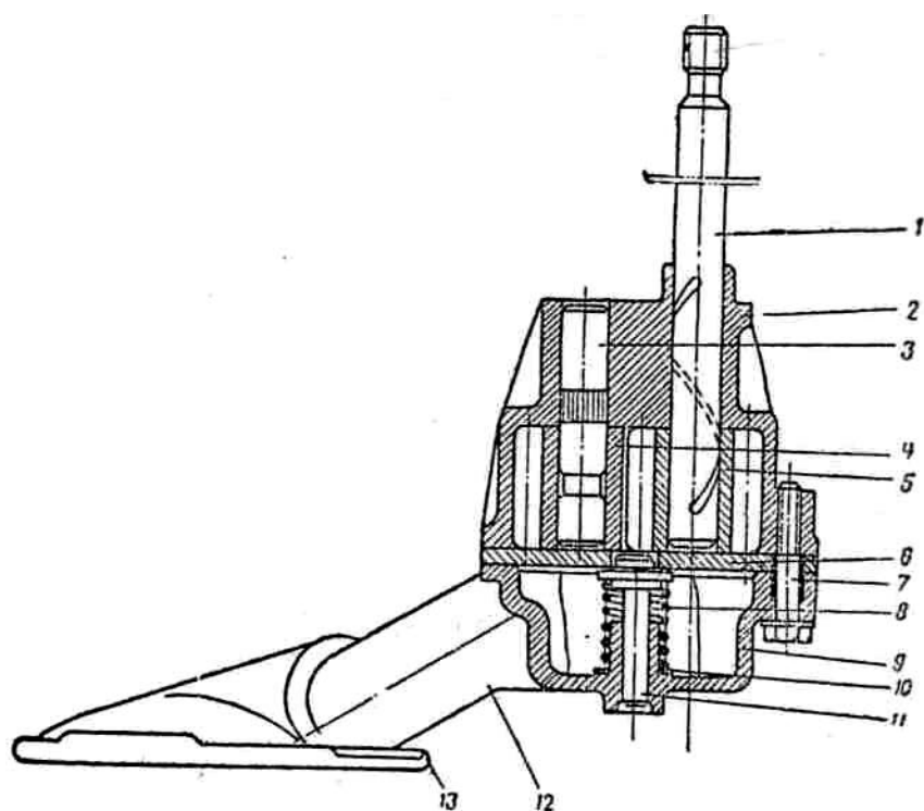
Рис.5. Масляный насос:
