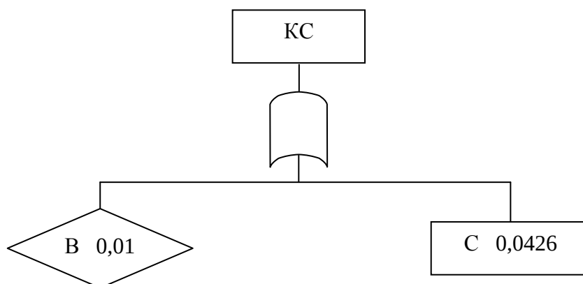
Рис. 3.2. Фрагмент «дерево причин» изображенное на рис. 2.2
