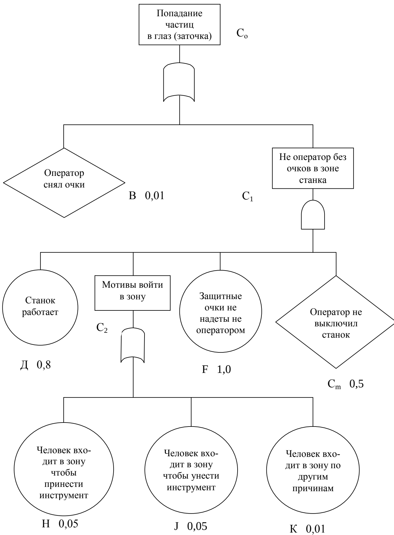
Рис.2.2. Логическая схема дерева причин
