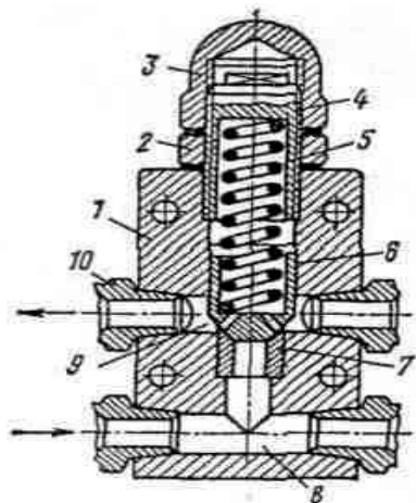
Рис.1. Предохранительный клапан: 1 – корпус, 2 – контргайка, 3 – колпак, 4 – винт, 5 – пружина, 6 – клапан, 7 – седло, 8, 9 – нагнетательный и сливной каналы, 10 – штуцер.
