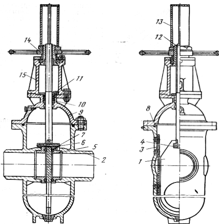
Рис. 17. Параллельная однодисковая задвижка:
