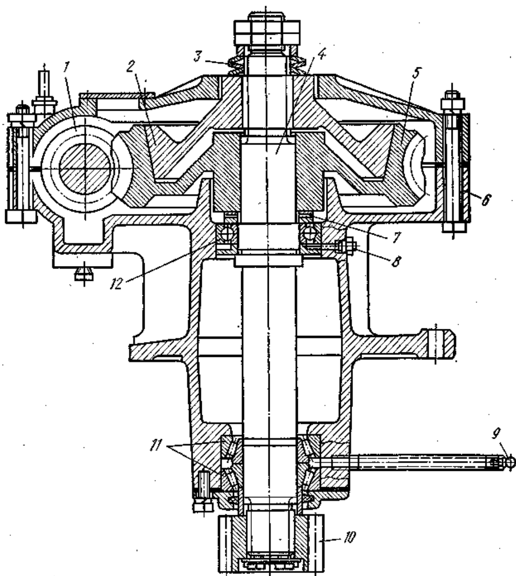
Рис. 32. Механизм поворот, крана КС-2561 Е с фрикционной предохранительной конической муфтой:
