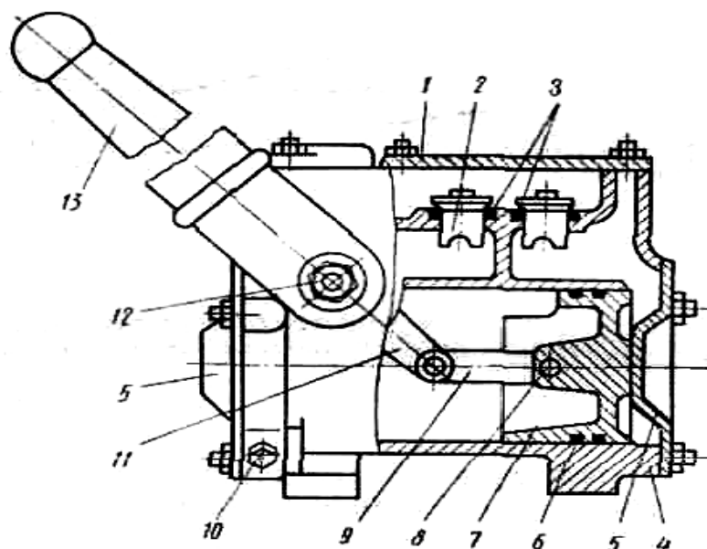
Рис. 8. Ручной одноцилиндровый поршневой насос двойного действия:
