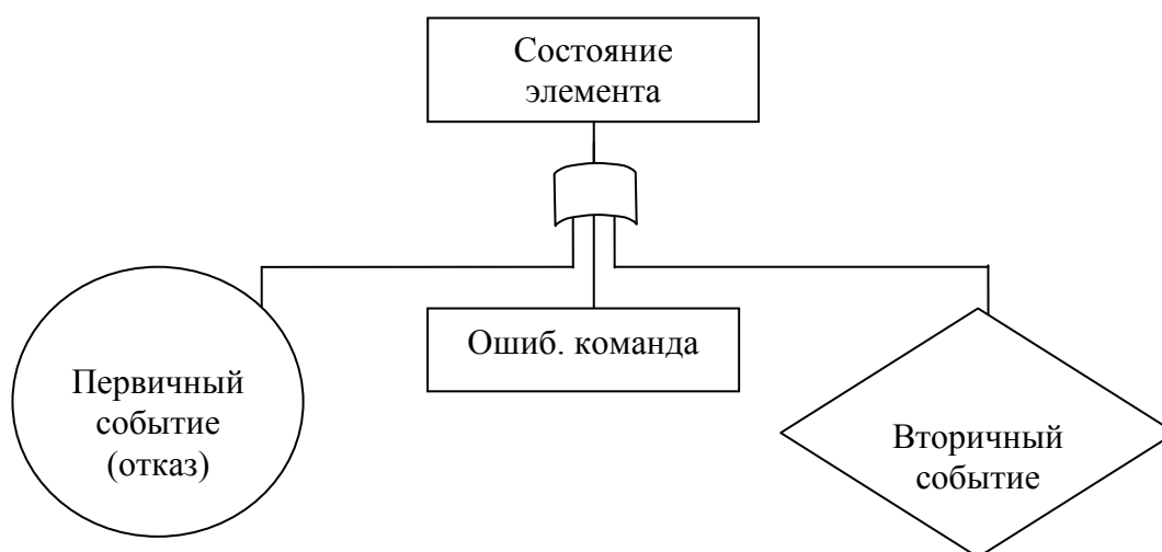
Рис. 2.1. Схема к построению «дерева отказов»
