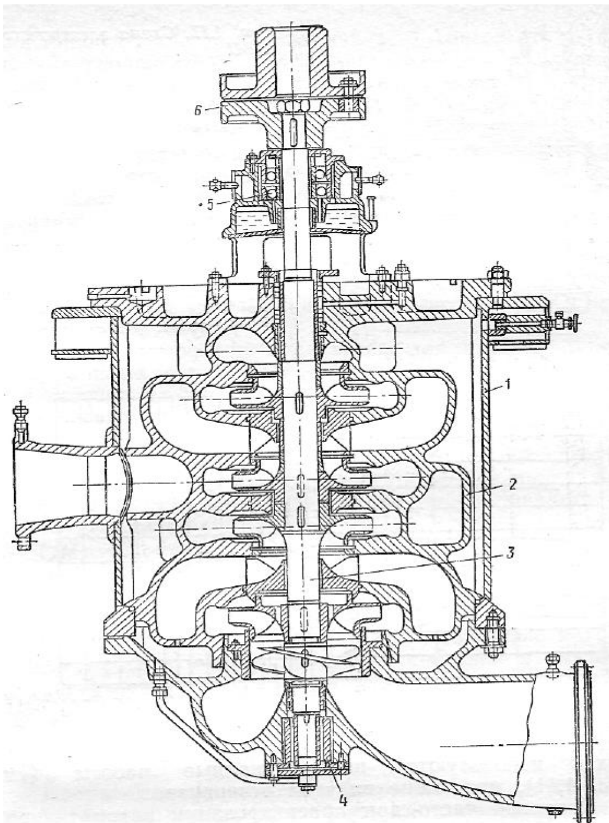
Рис. 29. Конденсатный насос:
