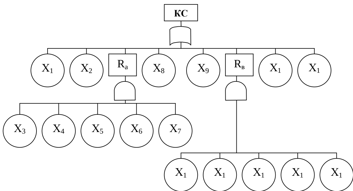
Рис. 6.4. «Дерево отказов»
