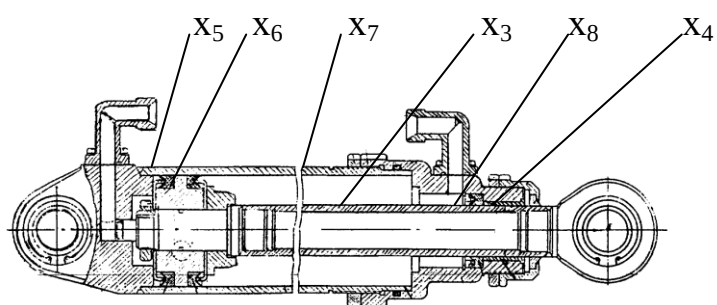
Рис. 6.1. Устройство для загибания тросов анкеров
