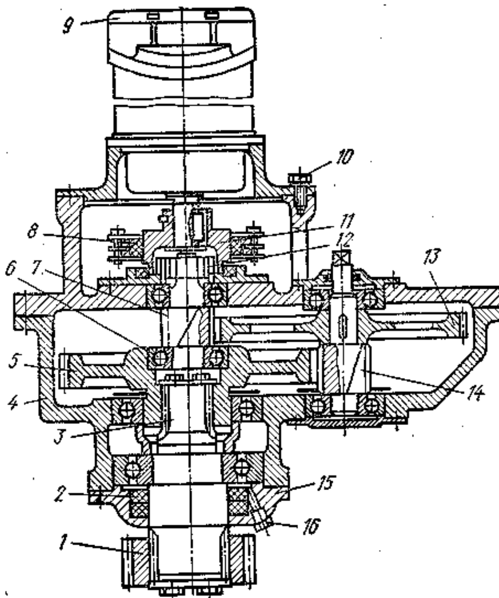
Рис. 7. Редуктор механизма поворота:
