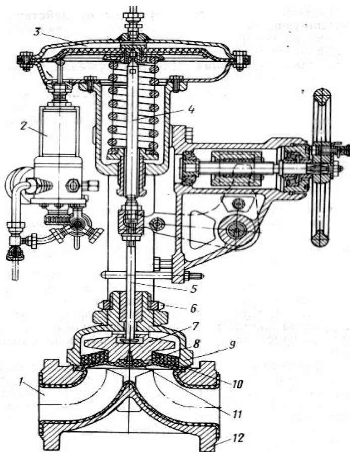
Рис. 15. Диафрагменный регулирующий клапан:
