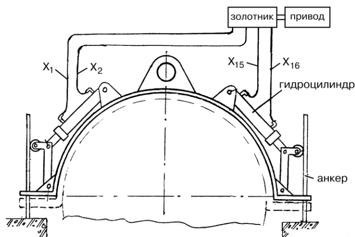
Рис. 6.1. Устройство для загибания тросов анкеров
