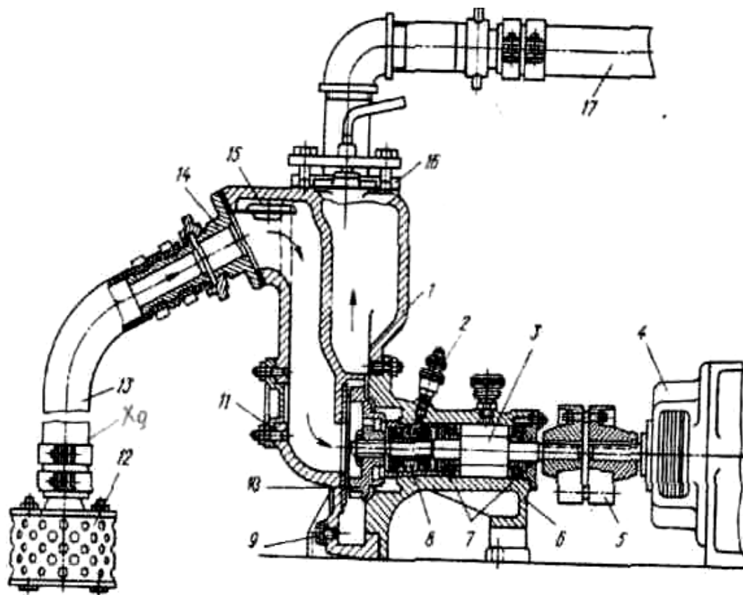
Рис.2. Самовсасывающий центробежный насос:
