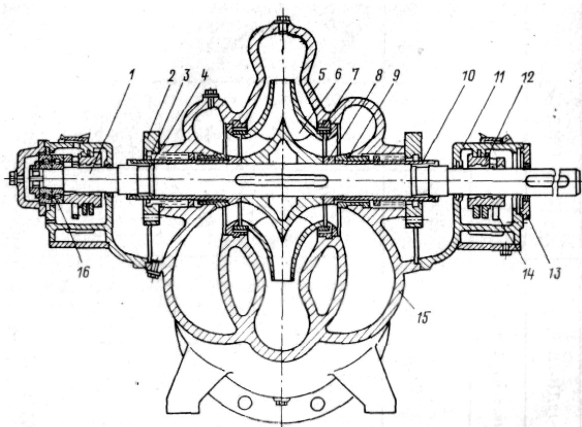
Рис. 24. Горизонтальный грузовой насос СН-56-30
