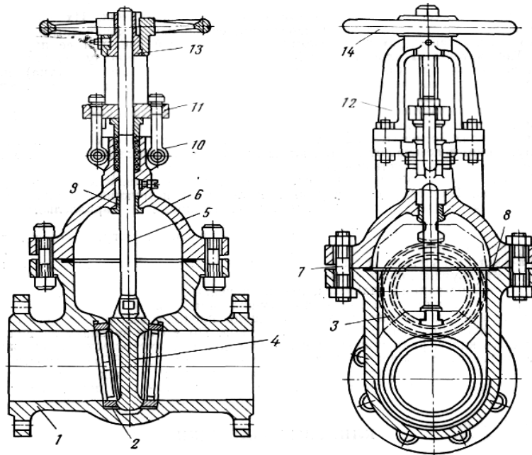
Рис. 18. Полнопроходная задвижка с цельным клином:
