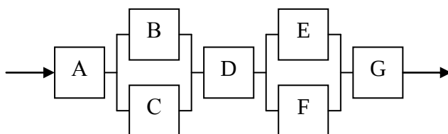
Рис. 5.3. Структурная схема системы
