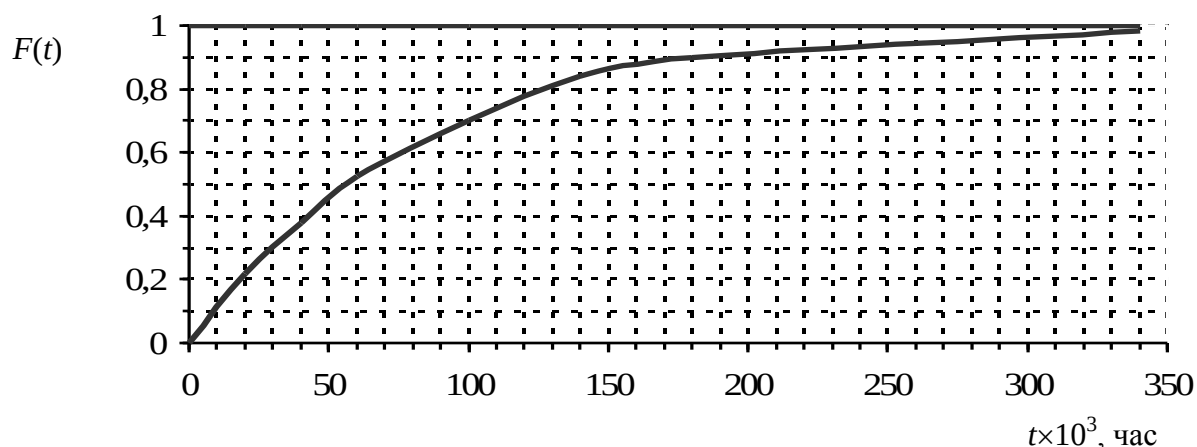
Рис. 6.5. Интегральная функция экспоненциального распределения, \lambda=1,25 \times 10^{-5} , 1/час.
