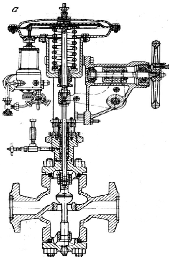
Рис. 14. Односедельный регулирующий клапан с мембранным исполнительным механизмом
