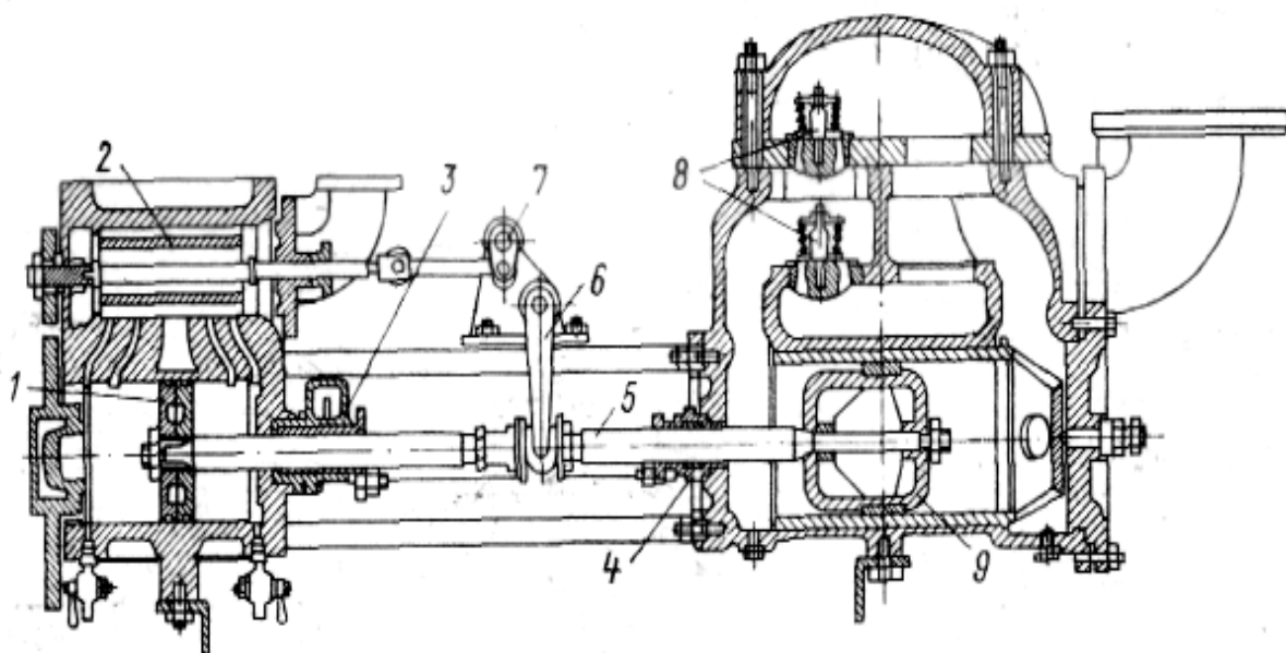
Рис. 20. Горизонтальный паровой насос:
