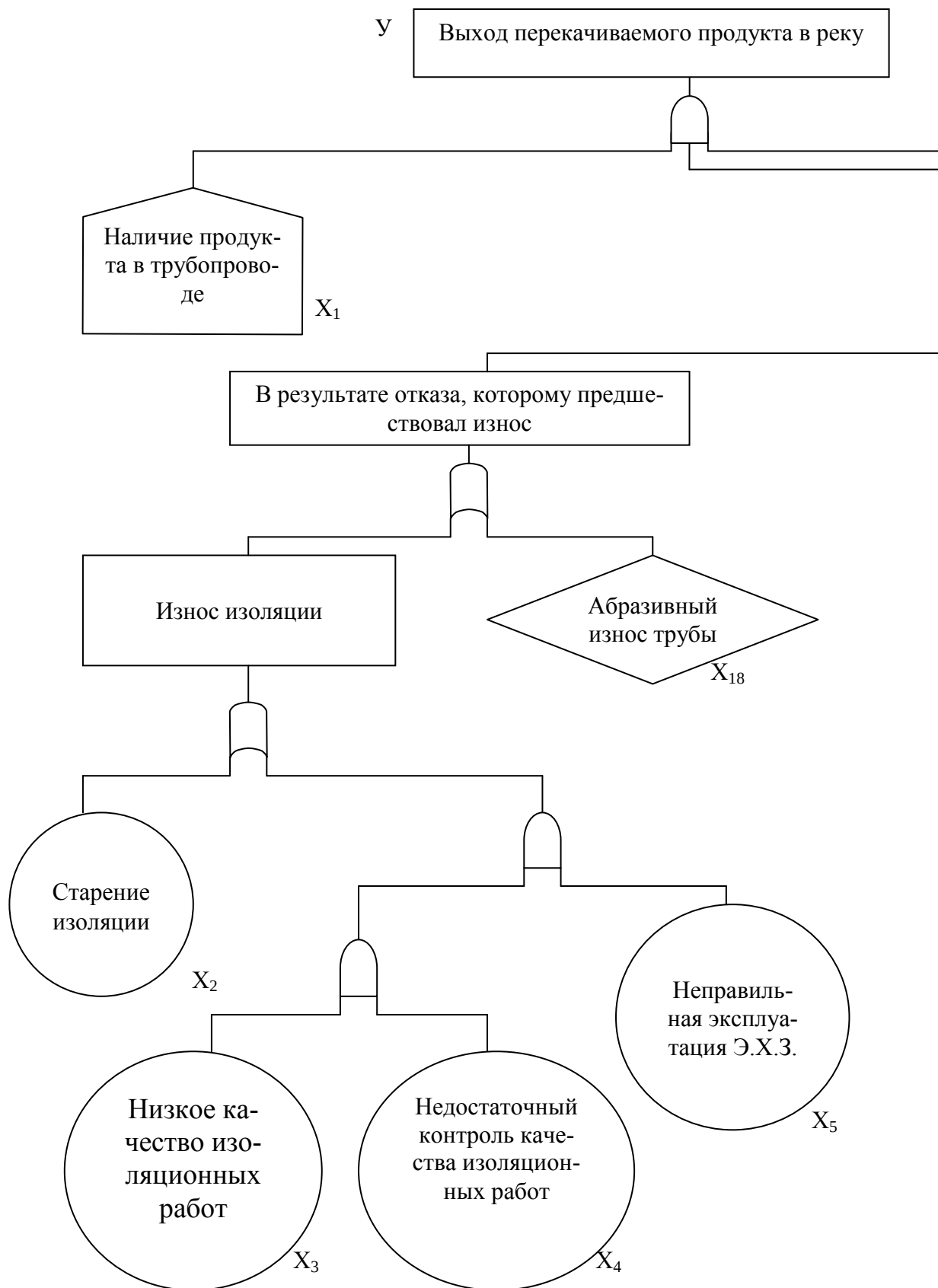
Рис. 4.2. «Дерево отказов» для предлагаемого
