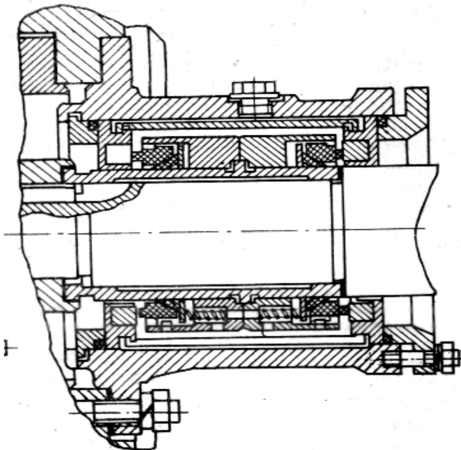
Рис.26. Торцовое двойное уплотнение
