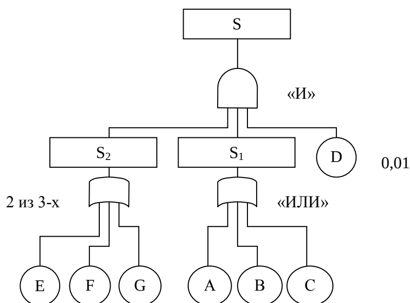
Рис. 5.1. «Дерево отказов» к примеру 1.
