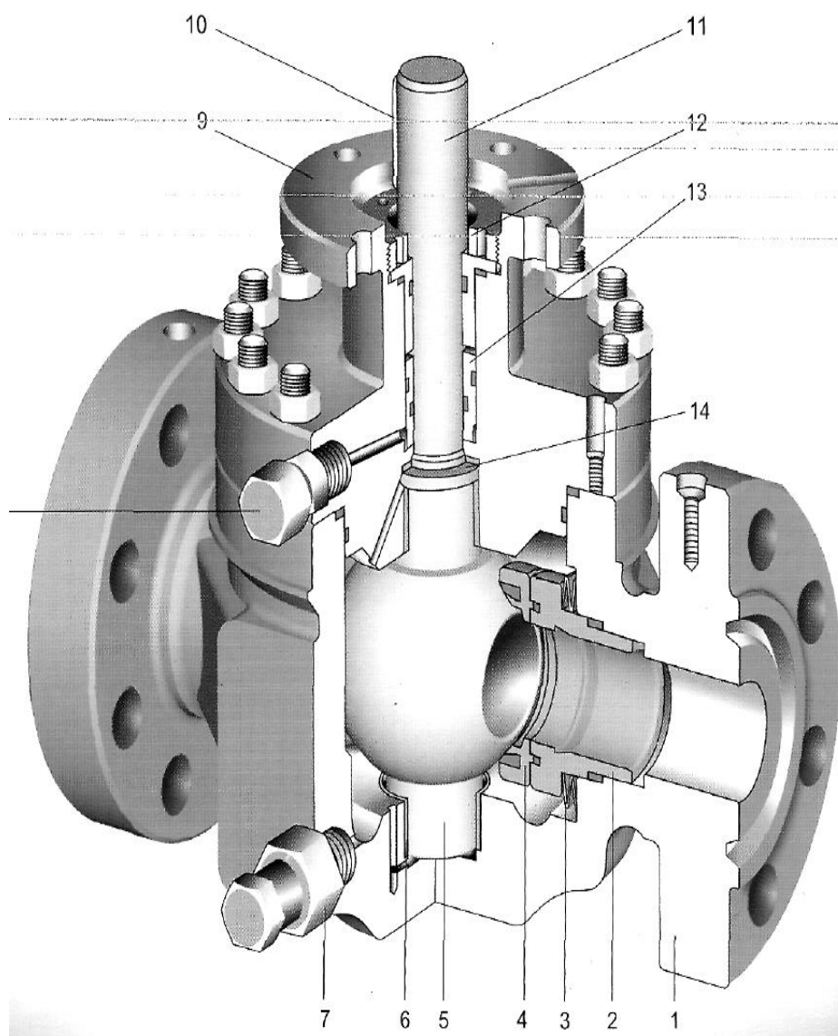
Рис. 31. Шаровой кран КШ-Р:
