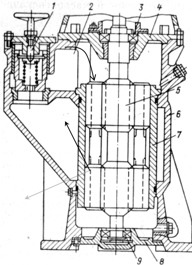
Рис. 23. Вертикальный трехвинтовой насос ЭМН 335/4,5
