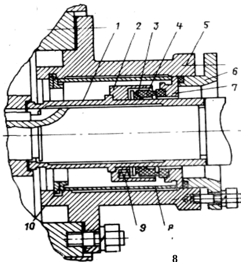
Рис. 25. Торцовое одинарное уплотнение
