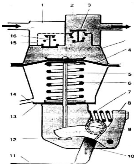
Рис.4. Топливный насос: 1 – всасывающая полость; 2 – нагнетательная полость; 3 – нагнетательный клапан; 4 – мембрана; 5 – шток мембраны; 6 – пружина; 7 – возвратная пружина приводного рычага; 8 – приводной рычаг; 9 – ось рычага ручной подкачки; 10 – возвратная пружина рычага ручной подкачки; 11 – рычаг ручной подкачки; 12 – головка штока; 13 – уплотнитель штока; 14 – дренажное отверстие; 15 – сетчатый фильтр; 16 – всасывающий клапан.
