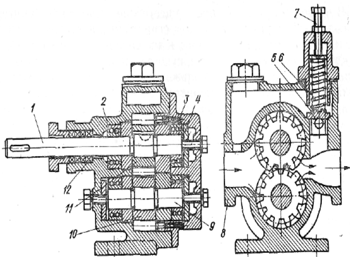
Рис. 27. Двухроторный насос с внешним зацеплением
