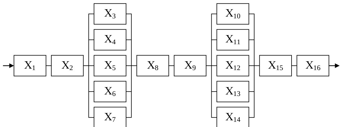
Рис. 6.3. Структурная схема надежности механической системы
