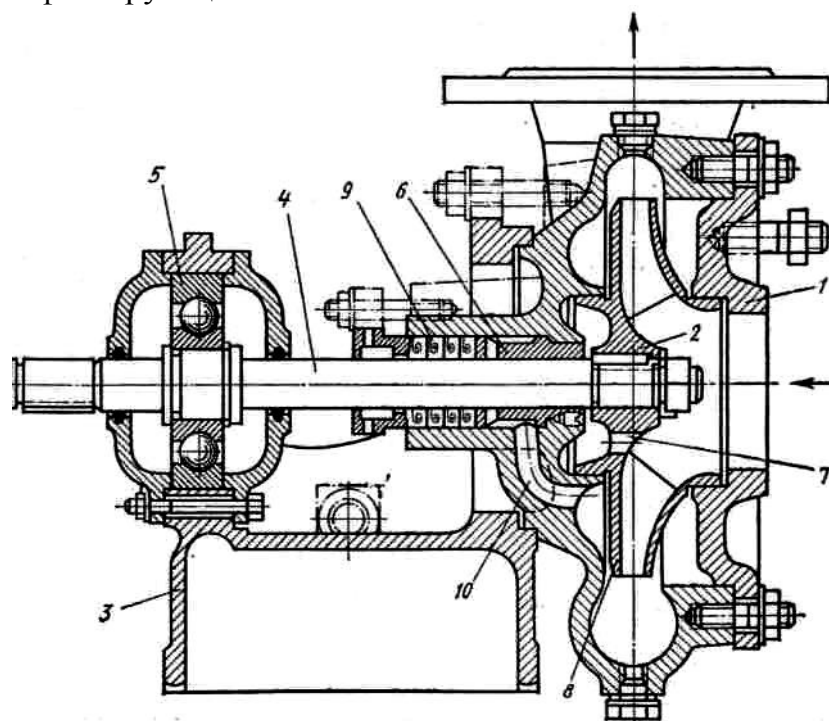
Рис.6. Центробежный насос ЦНШ одностороннего всасывания:
