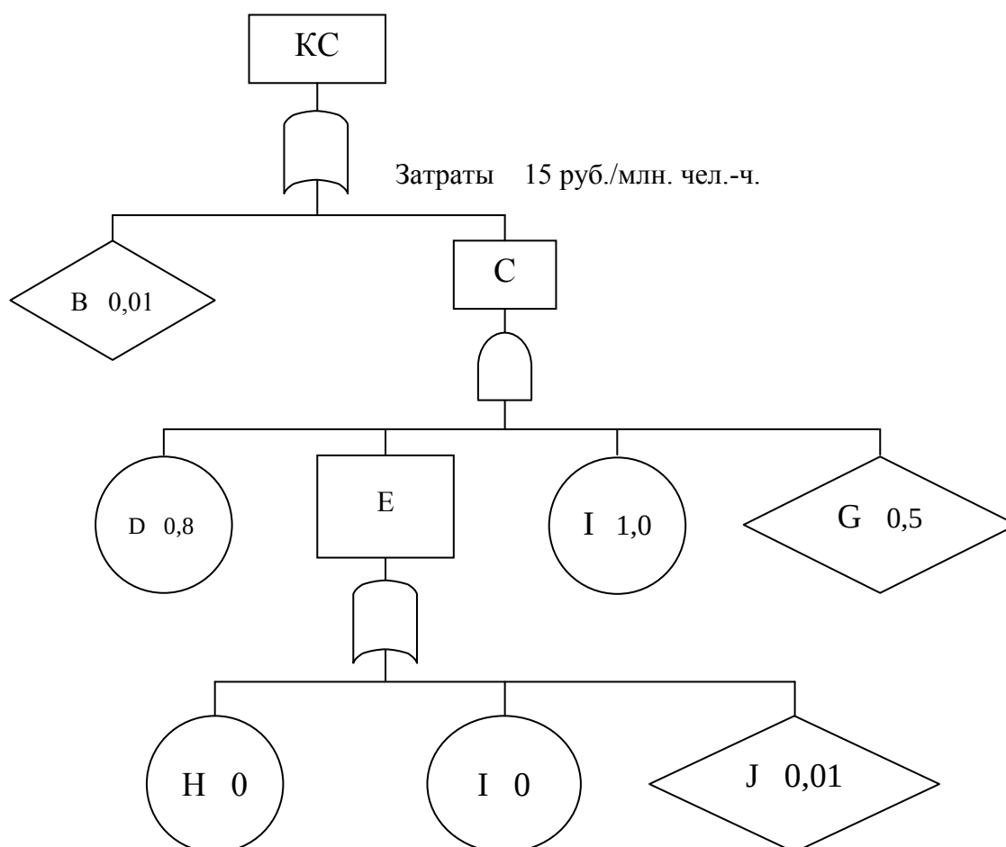
Рис.3.6 Дерево причин для альтернативы 3
