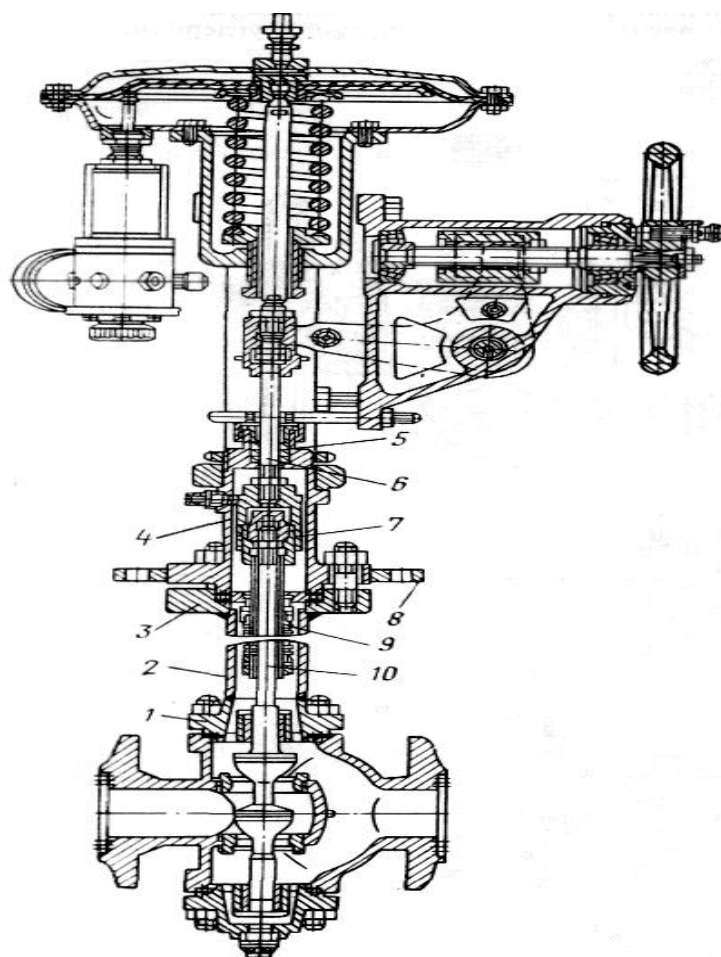
Рис. 13. Двухседельный сильфонный регулирующий клапан с пневматическим мембранным исполнительным механизмом:
