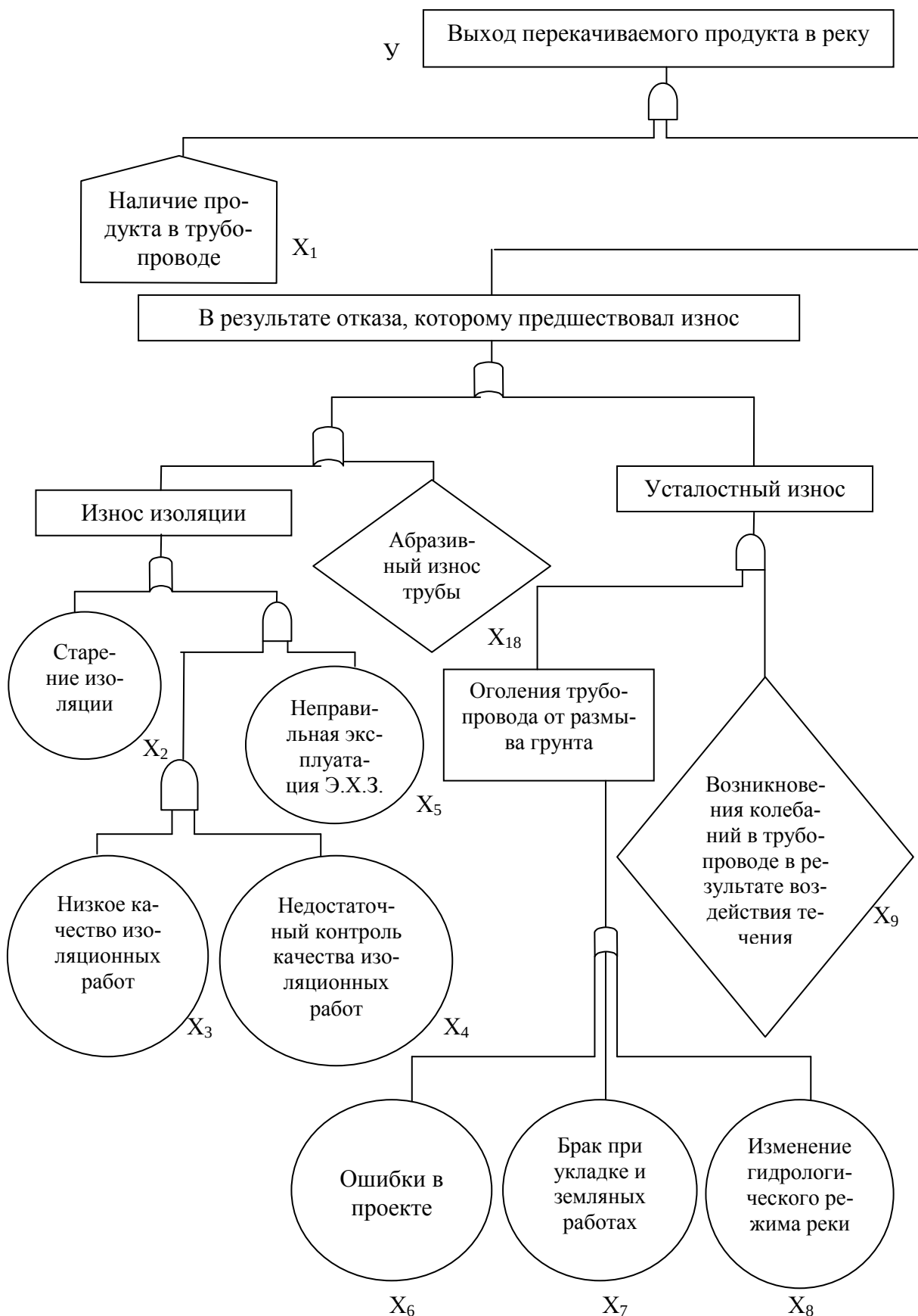
Рис. 4.1. «Дерево отказов» для традиционного
