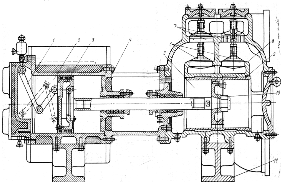
Рис. 19. Горизонтальный двухцилиндровый паровой прямодействующий насос
