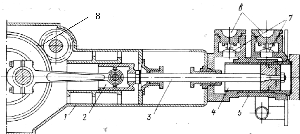
Рис. 21. Горизонтальный двухцилиндровый насос двухстороннего действия
