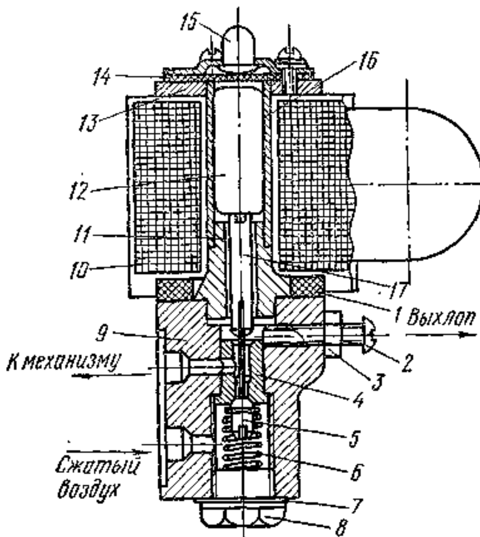
Рис. 9. Электропневматический вентиль ВВ-32Ш:
