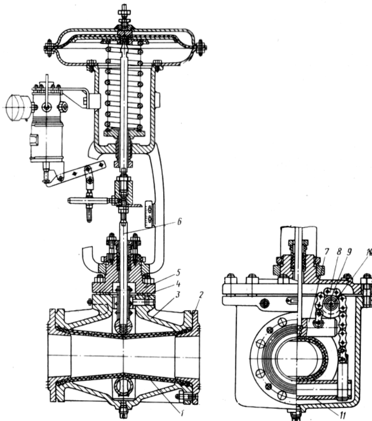
Рис. 16. Шланговый регулирующий клапан:
