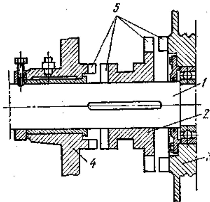
Рис. 33. Кулачковая муфта двустороннего действия: 1 – вал; 2 – подвижная полумуфта; 3 и 4 – правая и левая неподвижные полумуфты; 5 – кулачки.
