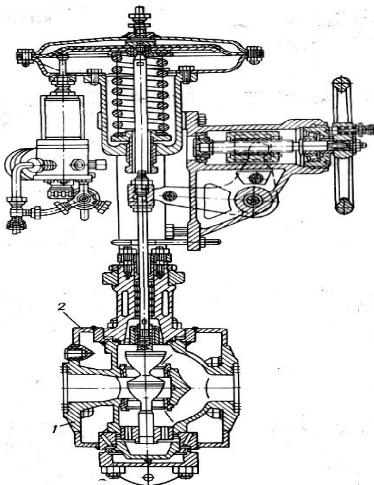
Рис. 12. Регулирующий двухседельный клапан с пневматическим мембранным исполнительным механизмом, рубашкой обогрева и сальниковым уплотнением штока
