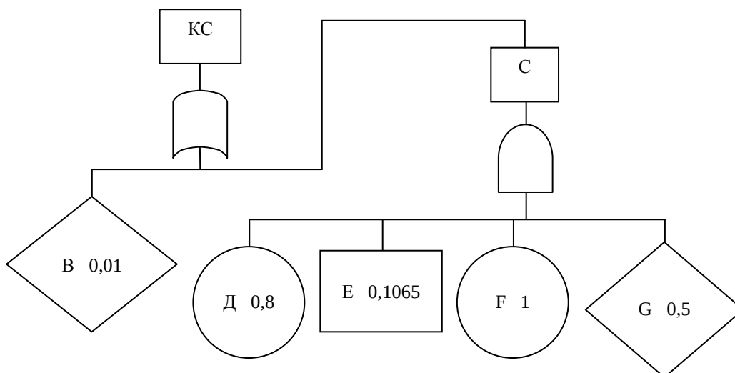
Рис. 3.1. Часть логической схемы «дерева причин» изображенной на рис.2.2
