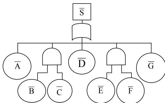
Рис. 5.4. Дерево отказов
