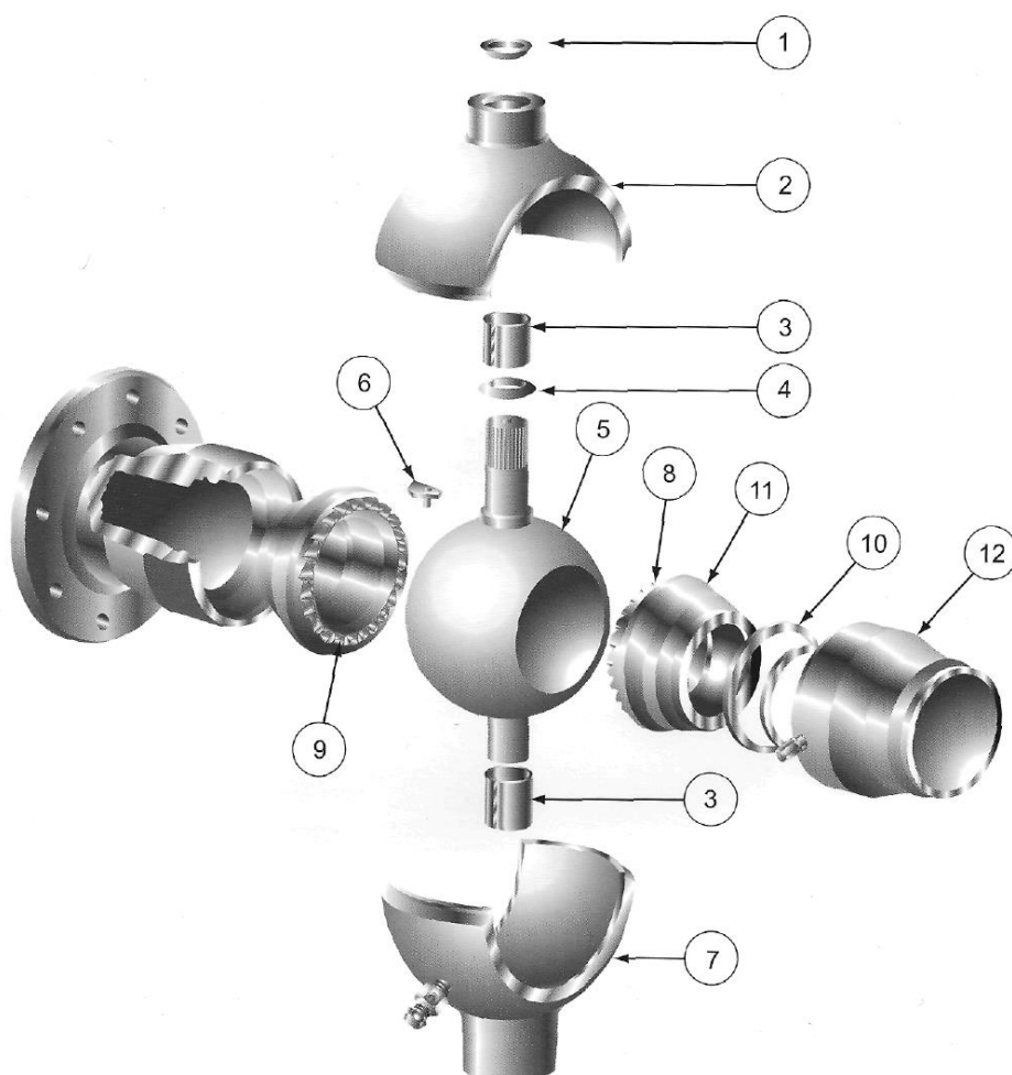
Рис. 28. Шаровой кран CBM:
