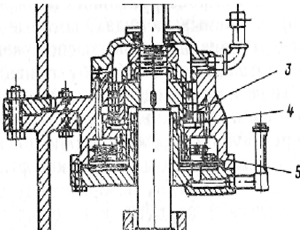
Рис. 30. Конденсатно-бустерный насос:
