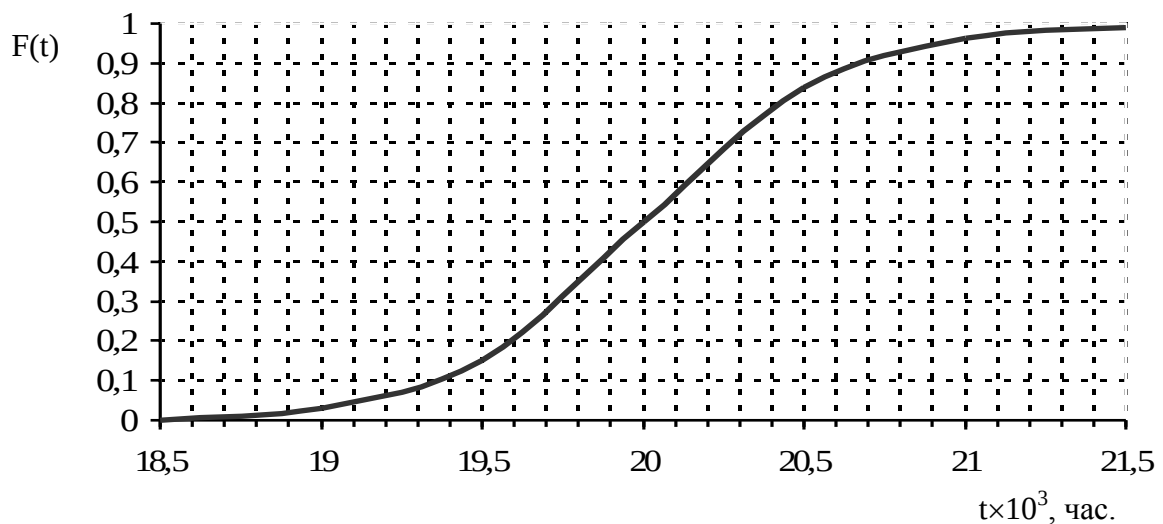
Рис. 6.7. Интегральная функция нормального распределения
