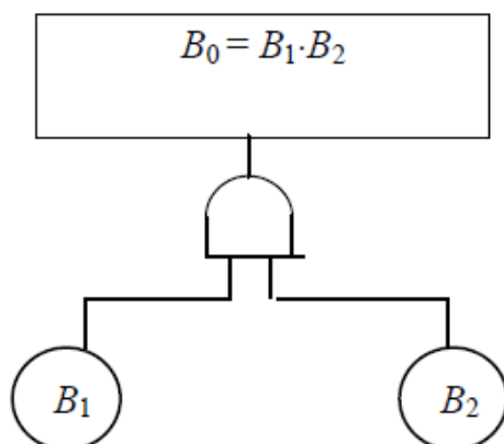
Рисунок 4.4 – Схема «И» с двумя входами
