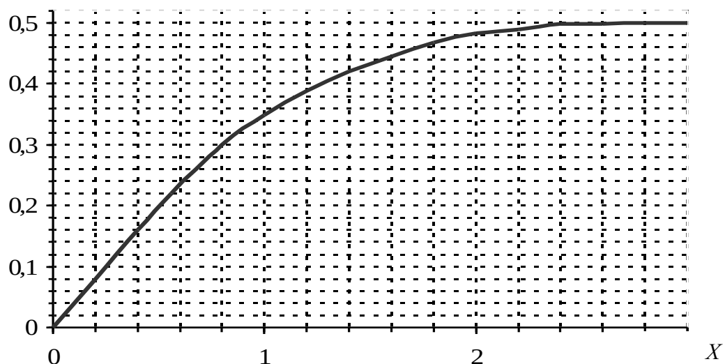
Рис. 6.6. Половинная функция Лапласа
