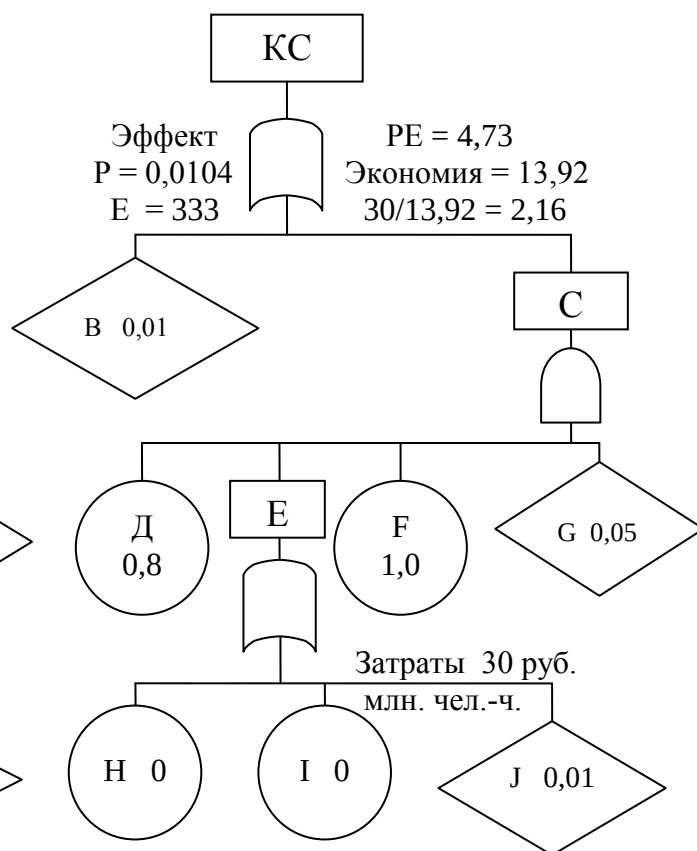
Рис.3.5 Дерево причин для альтернативы 2
