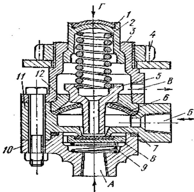
Рис. 10. Унифицированный пневмоклапан непрямого действия: 1 – чашка, 2 и 9 – пружины, 3 и 10 – крышки, 4 – гайка, 5 – стакан, 6 – диафрагма, 7 – уплотнение, 8 – клапан с уплотнителем, 11 – корпус, 12 – шайба.
