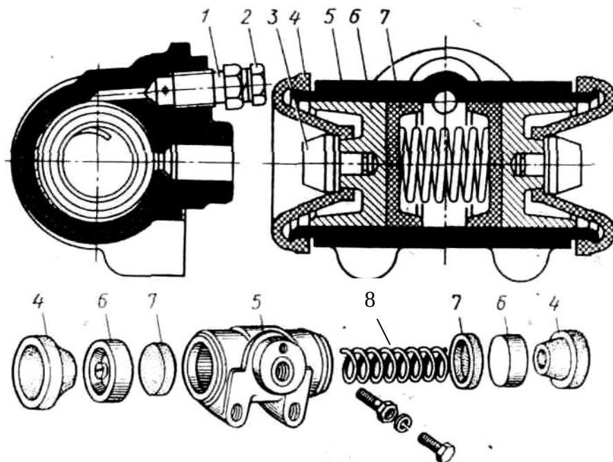
Рис.3. Тормозной цилиндр гидропривода (двухпоршневой): 1 – перепускной клапан; 2 – пробка; 3 – толкатель; 4 – резиновый чехол; 5 – корпус цилиндра; 6 – поршень; 7 – резиновая манжета; 8 – пружина.
