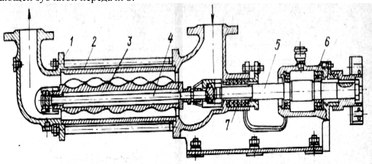
Рис. 22. Одновинтовой насос:
