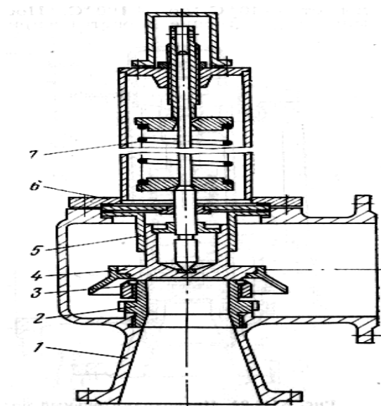
Рис. 11. Предохранительный клапан типа СППК4-200-16:
