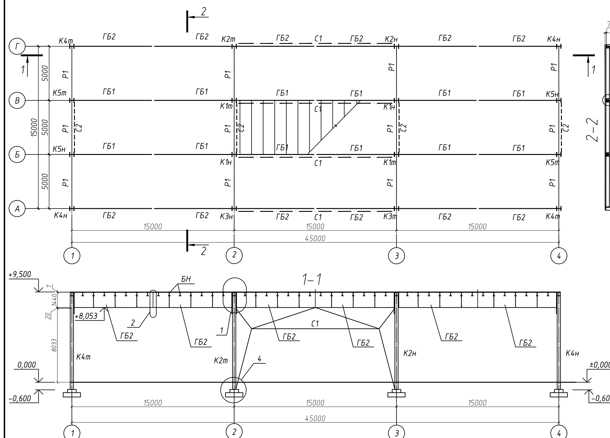
Монтажная схема рабочей площадки М1:200
