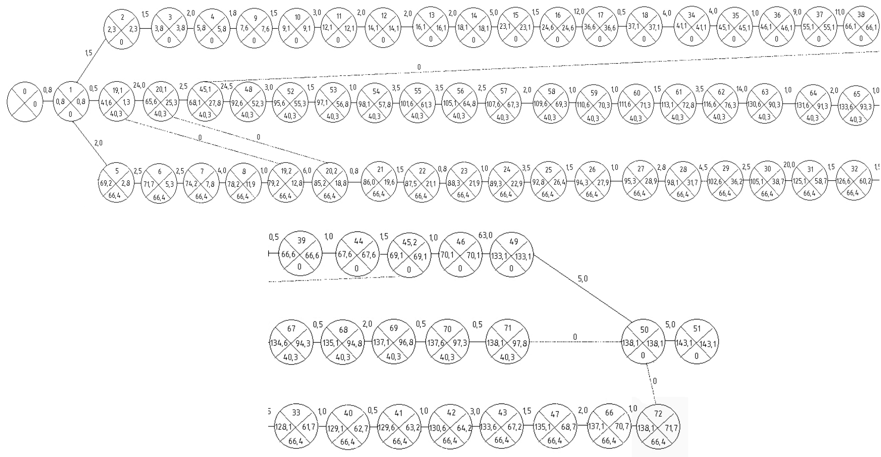
Рис. 4.3. Сетевой график технологического процесса ТО-1 автомобиля ВАЗ-21074
