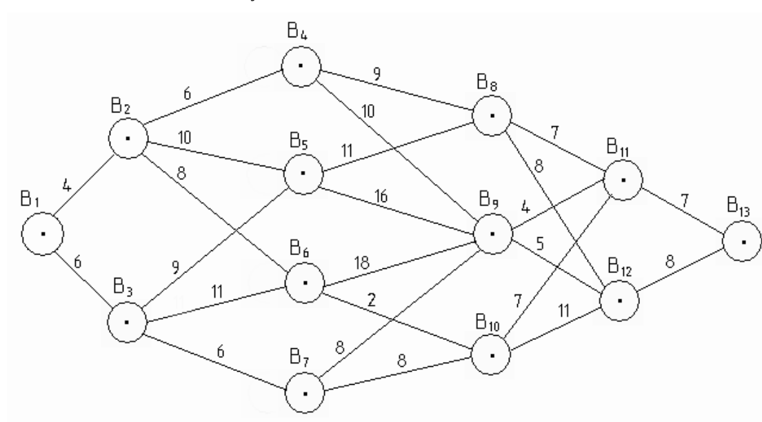
Рис. 2.2. Ориентированная сеть
