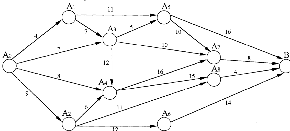
Рис. 2.5. Ориентированная сеть
