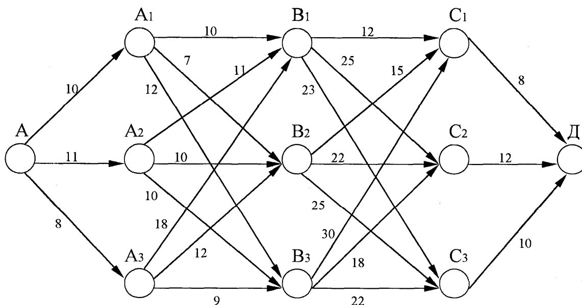
Рис. 2.7. Ориентированная сеть
