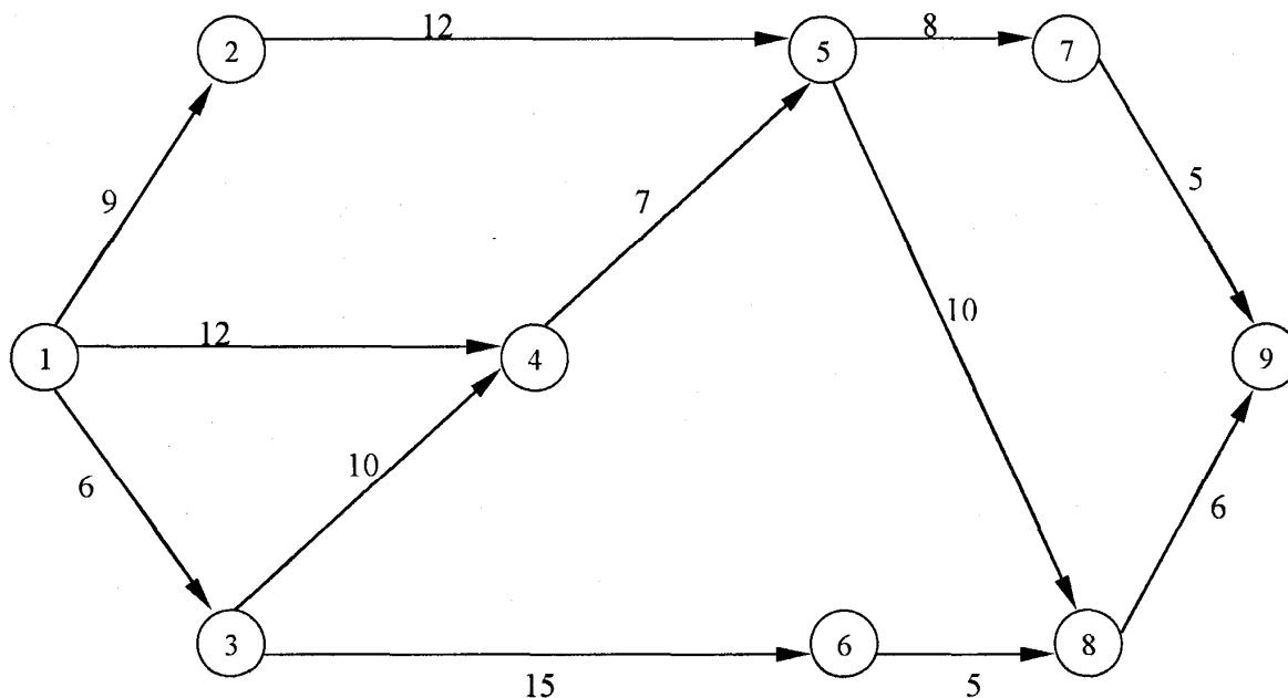
Рис. 4.10. Сетевой график
