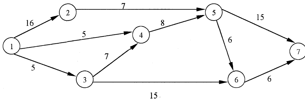
Рис. 4.4. Сетевой график
