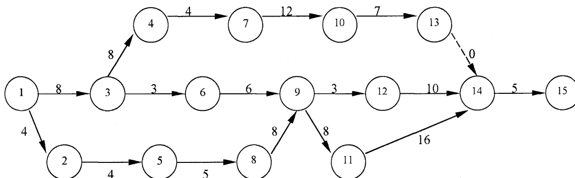
Рис. 4.8. Сетевой график
