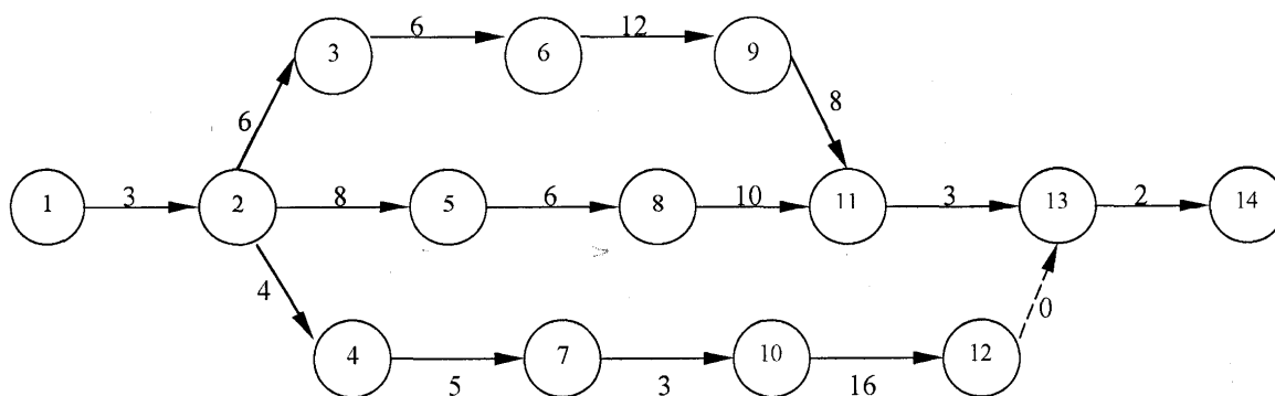
Рис. 4.7. Сетевой график
