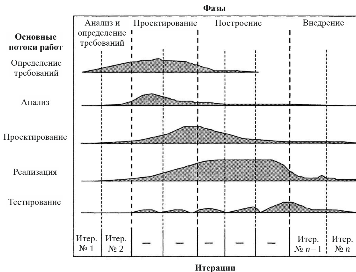
Рис. 3.3 – Модель RUP
