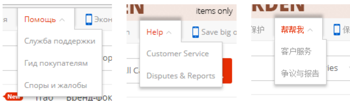
Рис. 4.5 – Пример локализации
