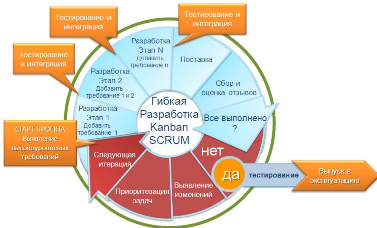
Рис. 3.4 – Гибкие модели
