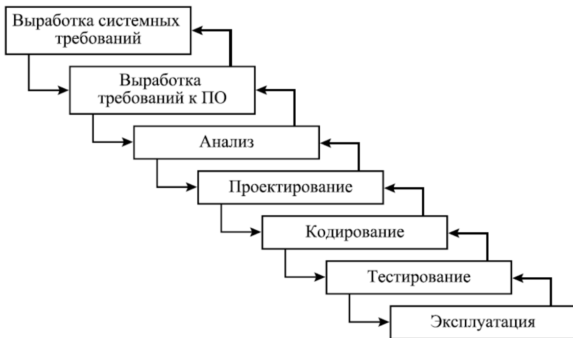
Рис. 3.1 – Водопадная модель
