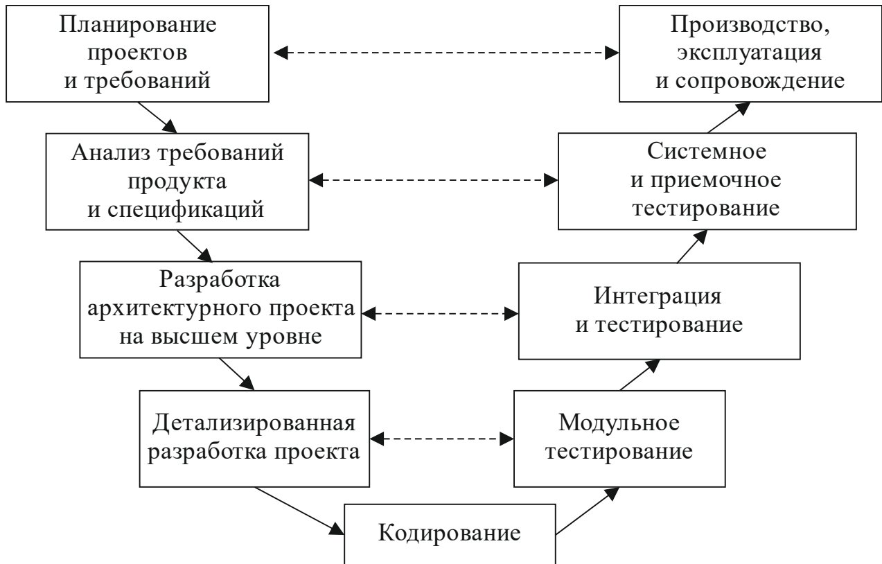
Рис. 3.2 – V-образная модель
