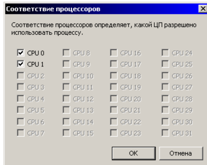
Рисунок 1.2 – Соответствие процесса и процессоров
