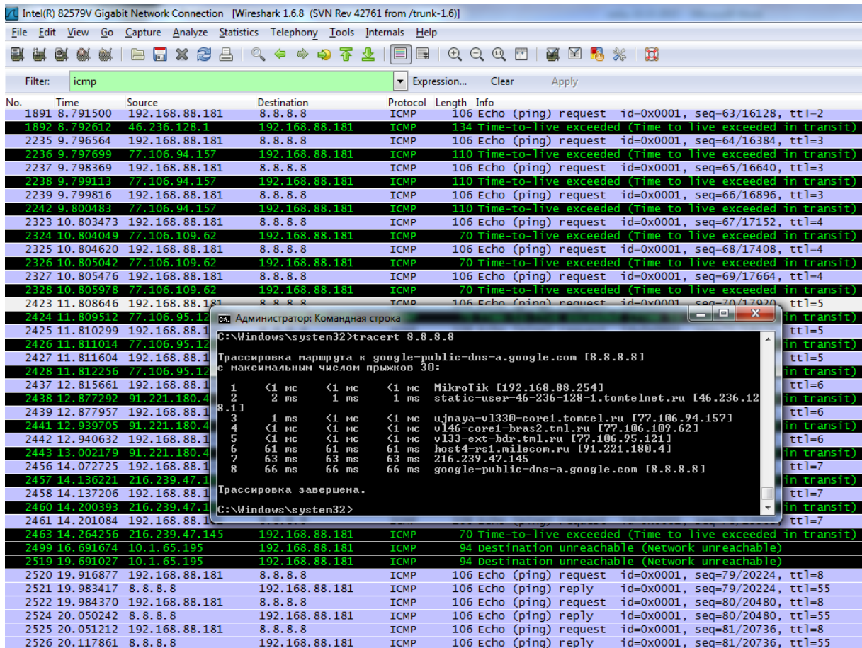
Рис. 2.5 – Результат выполнения команды tracert
