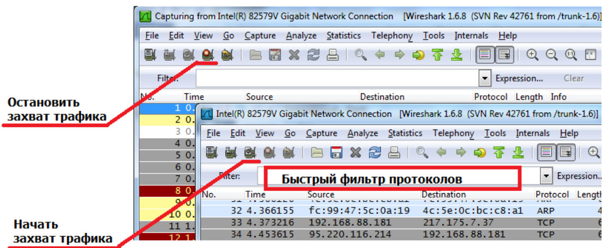
Рис. 2.2 – Захват трафика и быстрый фильтр
