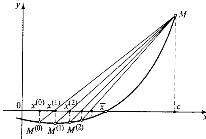
Рис. 3.5 – Метод ложного положения (общий случай)
