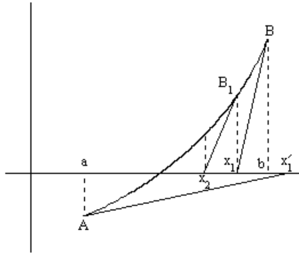
Рис. 3.2 – Геометрическая интерпретация метода Ньютона
