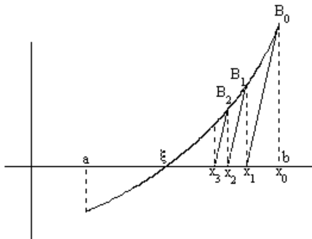
Рис. 3.4 – Модифицированный метод Ньютона
