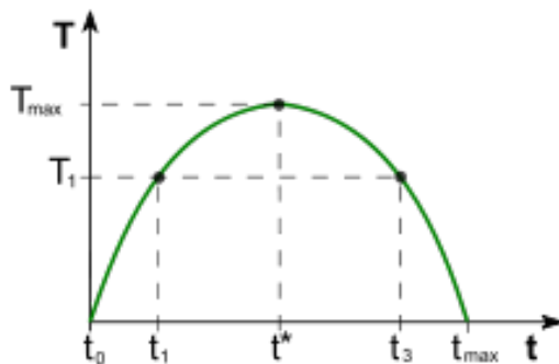
Рис. 2.1 – Кривая Лаффера
