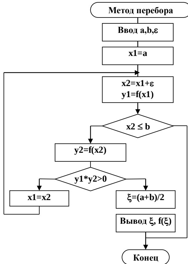
Рис. 1.3 – Схема алгоритма метода перебора
