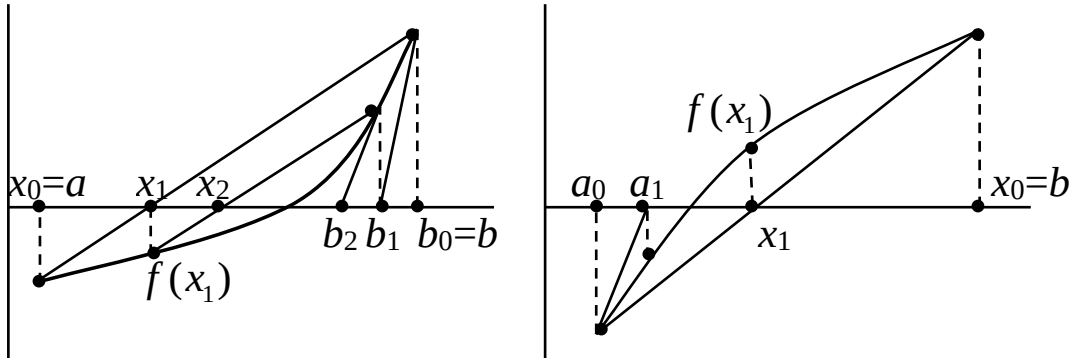
Рис. 1.12 – Геометрическая интерпретация комбинированного метода
