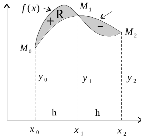
Рис. 5.2 – Геометрическая интерпретация формулы Симпсона
