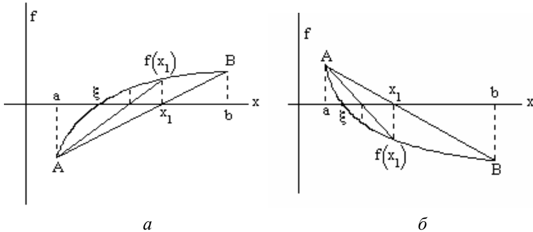
Рис. 1.6 – Графическая иллюстрация метода хорд (конец a неподвижен)
