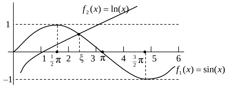
Рис. 1.1 – Графический метод решения уравнения f(x) = \ln x - \sin x
