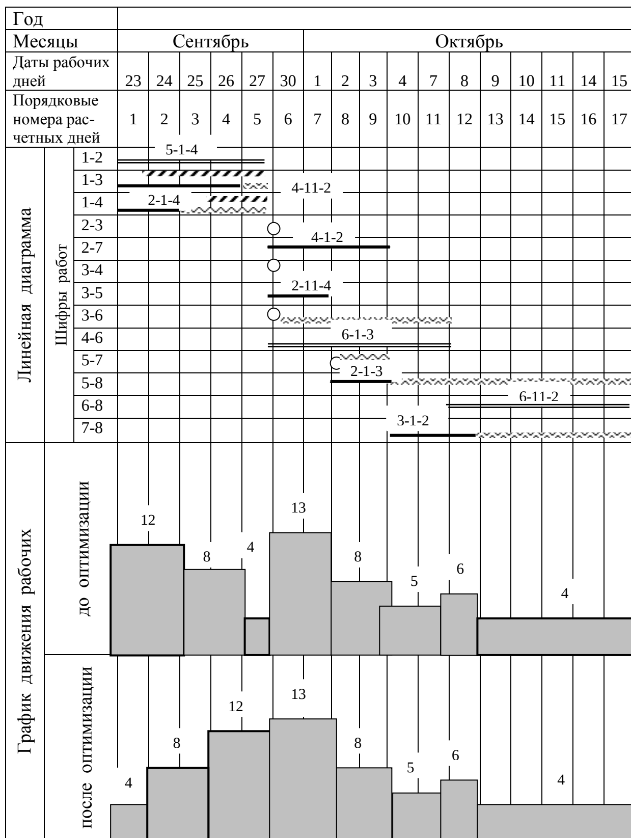
Рисунок 4.2 – Построение линейной диаграммы и эпюры трудовых ресурсов (первый вариант оптимизации)
