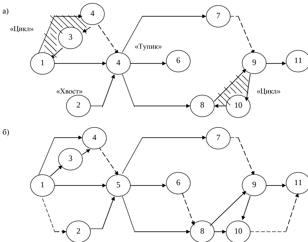
Рисунок 2.7 - Пример неправильного построения сети с «тупиками», «хвостами» и «циклами»:
