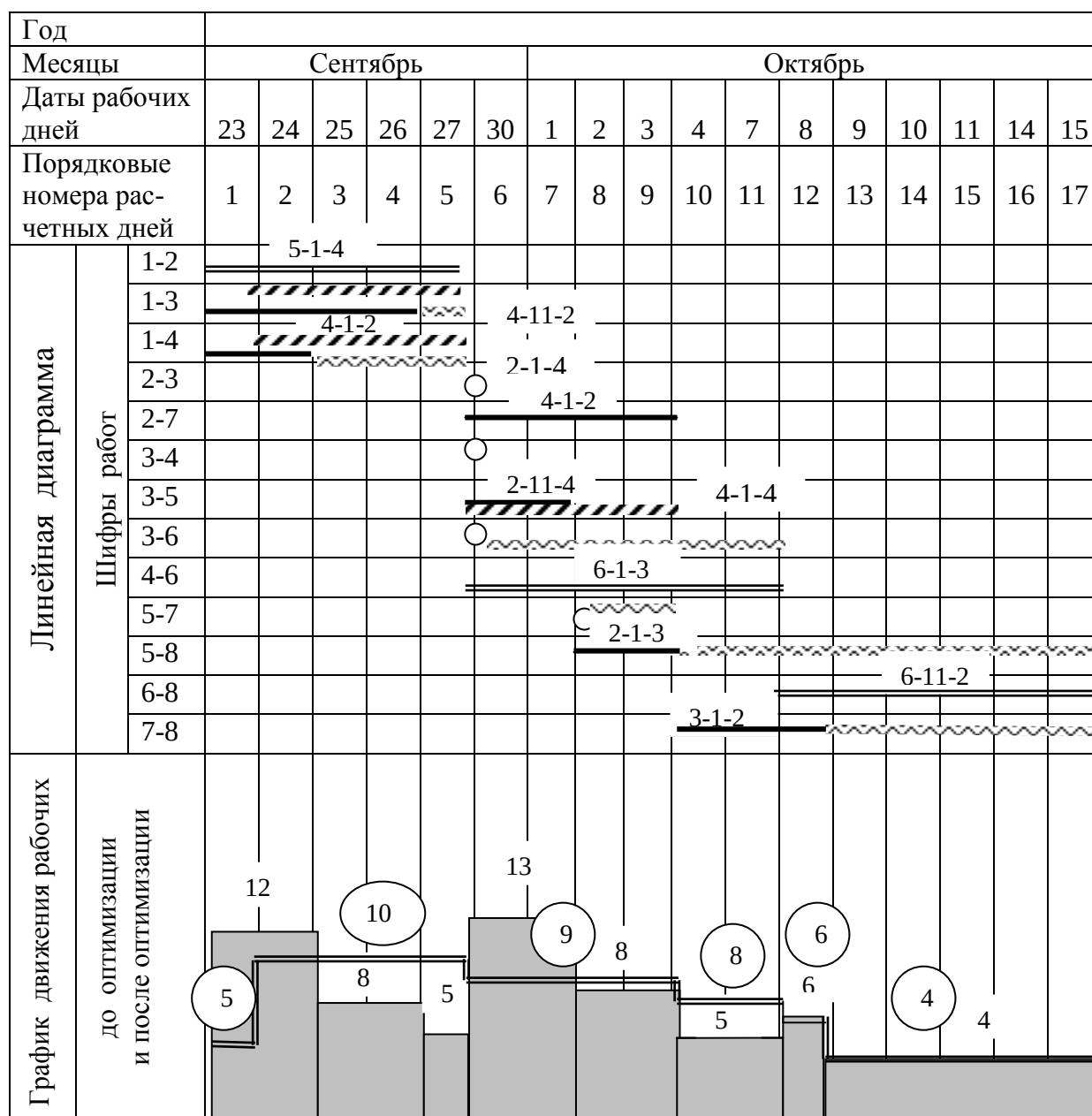
Рисунок 4.4 – Построение линейной диаграммы и совмещенных эпюр графиков движения трудовых ресурсов (второй вариант оптимизации)
