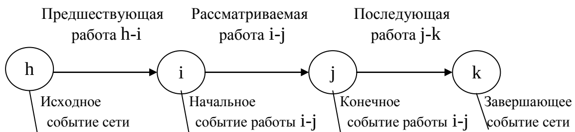
Рисунок 1.4 - Общая схема кодирования работ и событий сетевого графика
