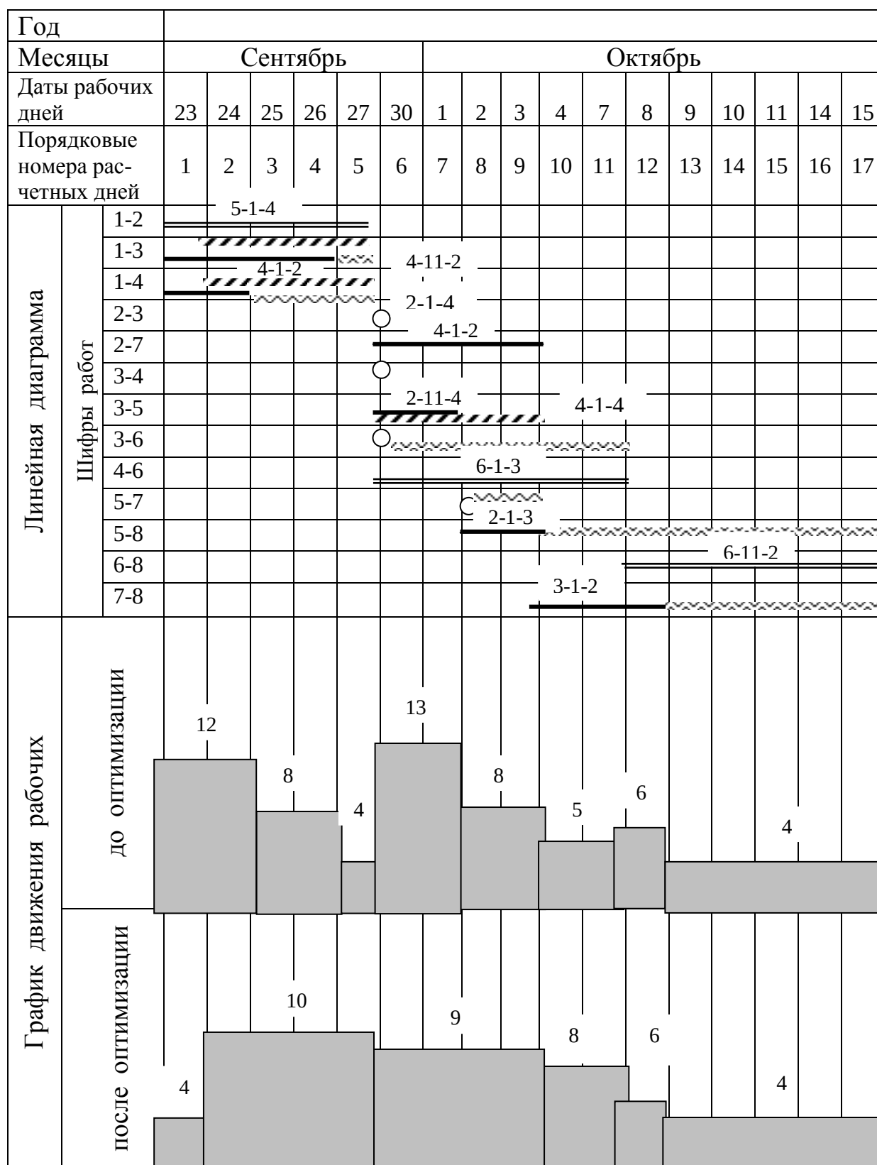
Рисунок 4.3 – Построение линейной диаграммы и эпюры трудовых ресурсов (второй вариант оптимизации)
