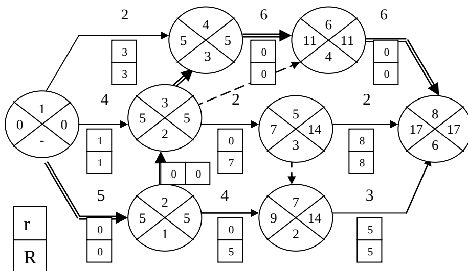
Рисунок 3.3 – Расчет сетевого графика графическим методом
