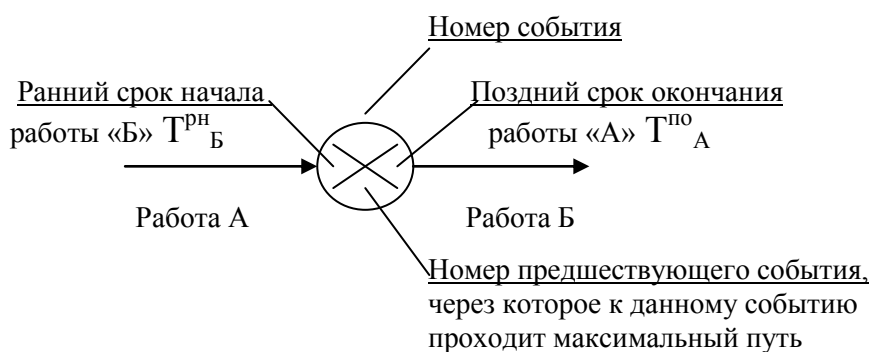
Рисунок 3.2 - Содержание секторов событий при расчете сетевого графика графическим методом
