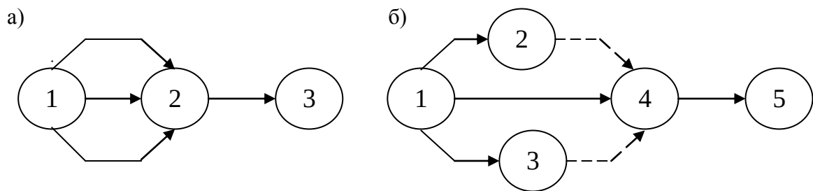
Рисунок 2.2 - Изображение параллельно выполняемых работ: а - неправильное; б - правильное
