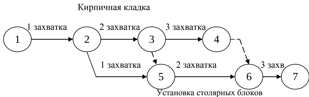
Рисунок 2.3 - Разбивка работ на части
