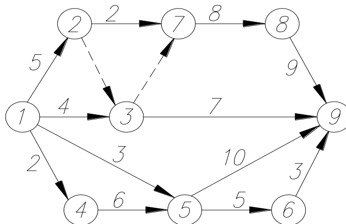
Рисунок 2.1 – сетевой график
