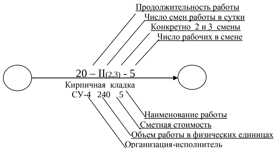
Рисунок 1.1 - Характеристики действительной работы
