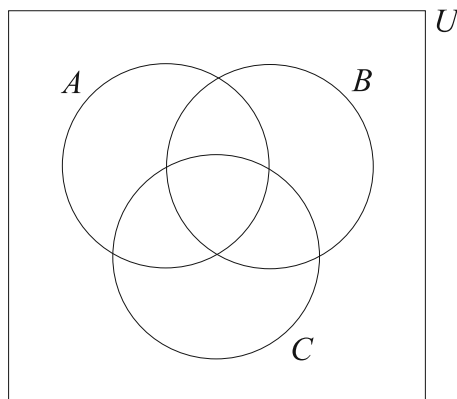
Рис. 3.3 – Диаграмма Венна для трех множеств
