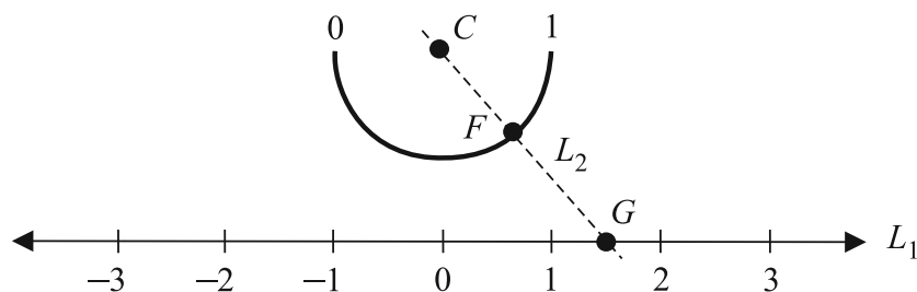
Рис. 3.9 – Полуокружность равномощна всей прямой
