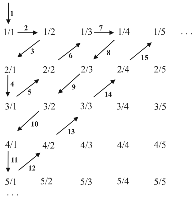
Рис. 3.11 – Множество \mathbb{Q} счётно
