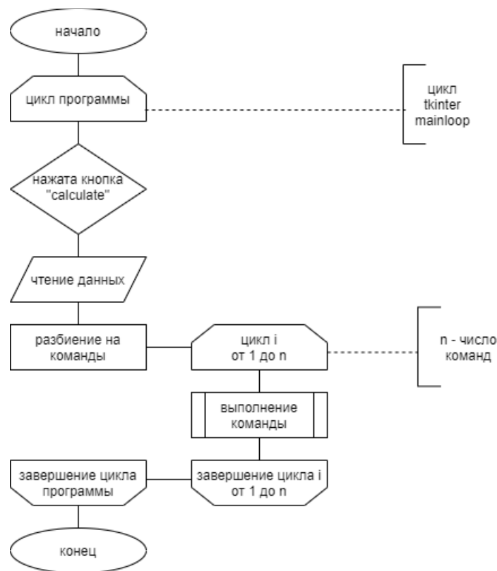
Рисунок 3 – блок схема алгоритма для второго задания
