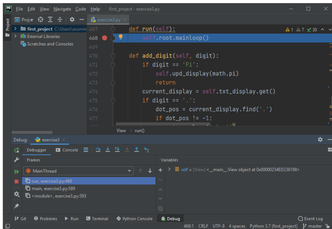
Рисунок 11 – Среда разработки в режиме отладки
