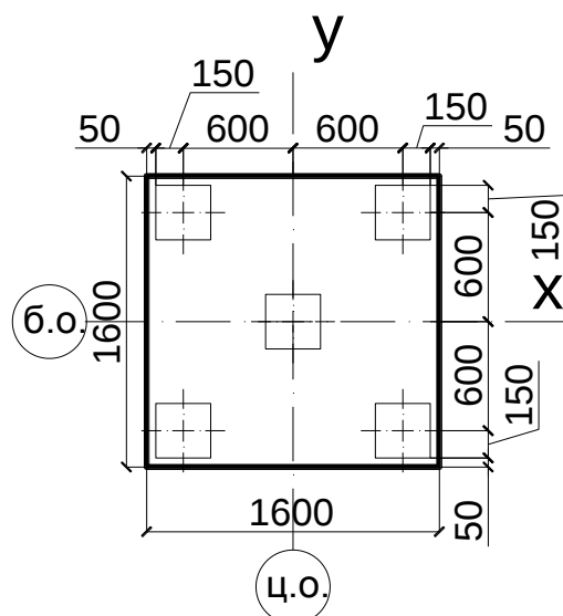
Рис. 13. Конструирование ростверка
