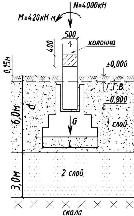
Рис. 2. Нагрузки на колонну по оси А и схема напластования грунтов
