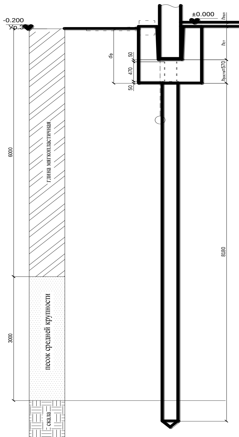
Рис. 11. Назначение конструктивной глубины заложения ростверка и длины сваи
