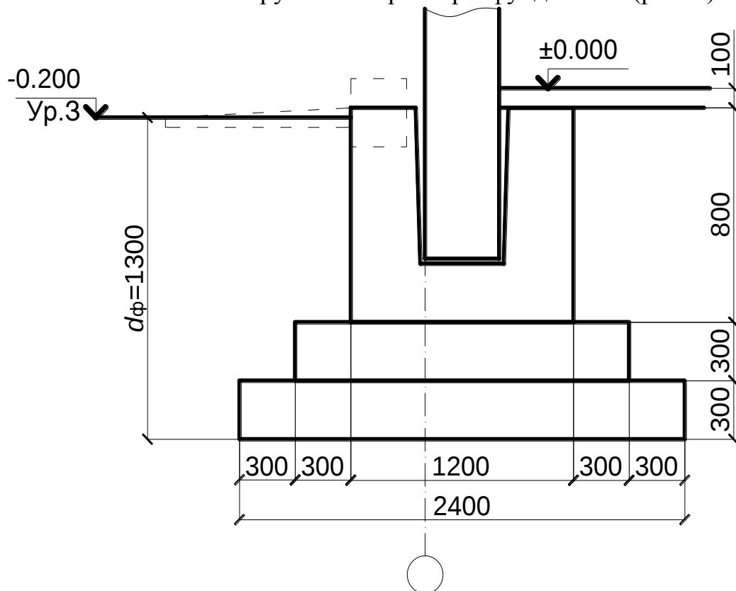
Рис. 4. Конструктивное решение фундамента
