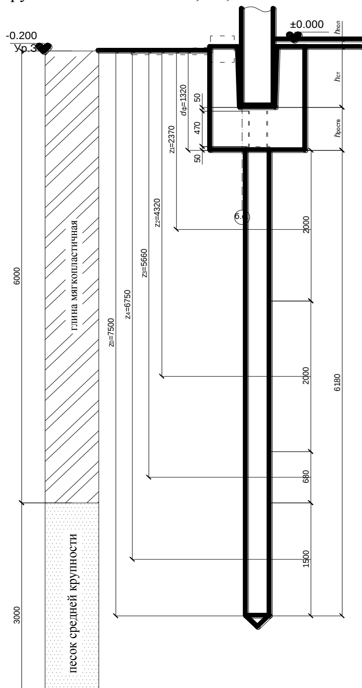
Рис. 8. Назначение конструктивной глубины заложения ростверка и длины свай
