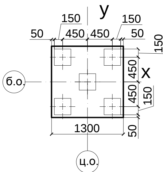
Рис. 12. Конструирование ростверка
