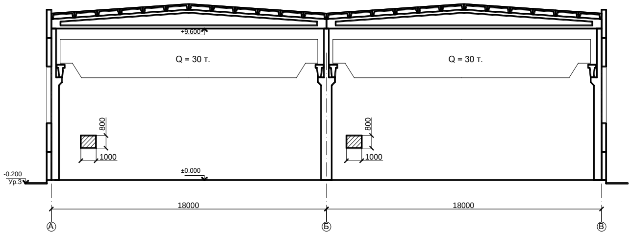
Рис. 1. Разрез здания
