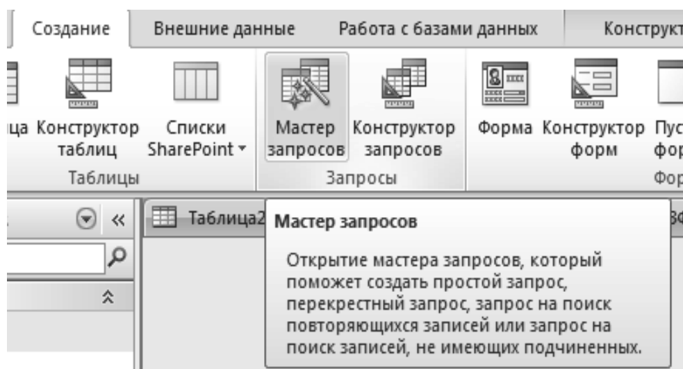
Рис. 2.19 — Панель «Запросы»
