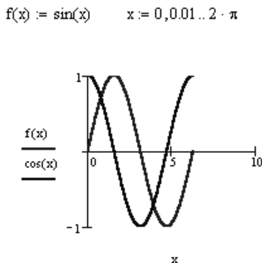
Рис. 4.35 – Функция f(x)
